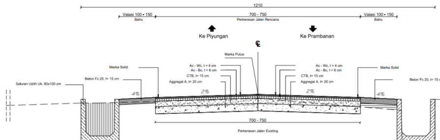
Gambar 3. 1 Potongan Melintang Jalan
