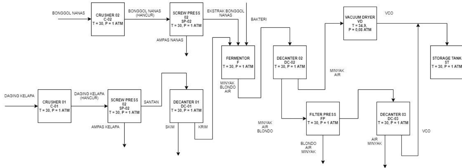
Gambar 4.4 Diagram Alir Kualitatif
