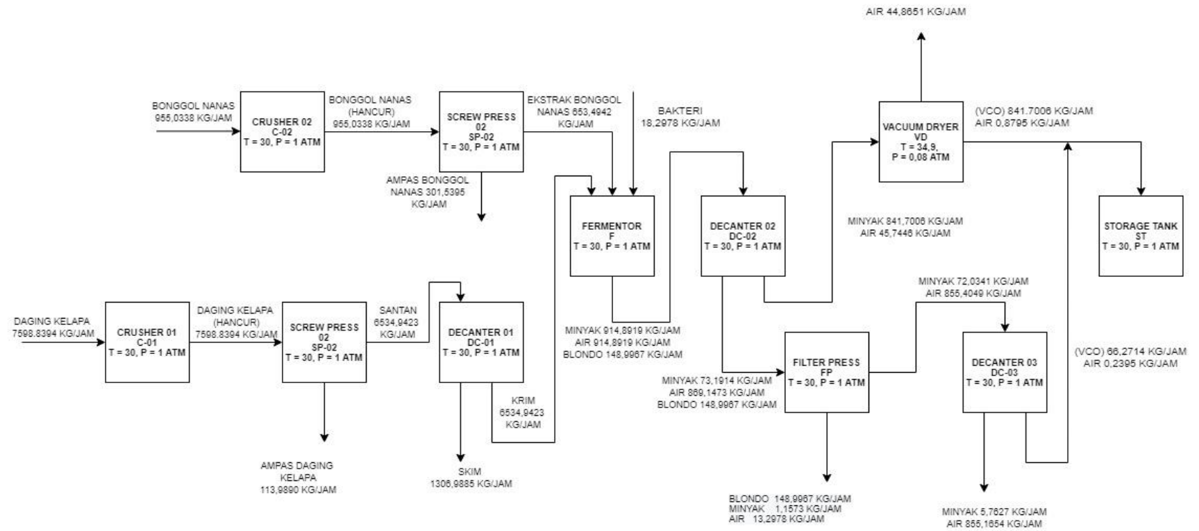
Gambar 4.3 Diagram Alir Kuantitatif
