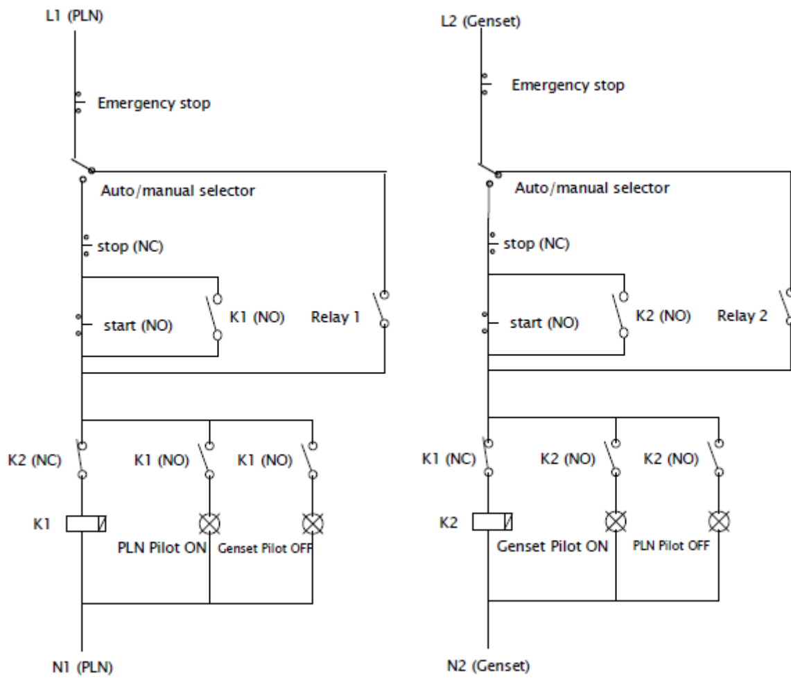
Gambar Diagram kendali PLN (kiri) dan genset (kanan)
