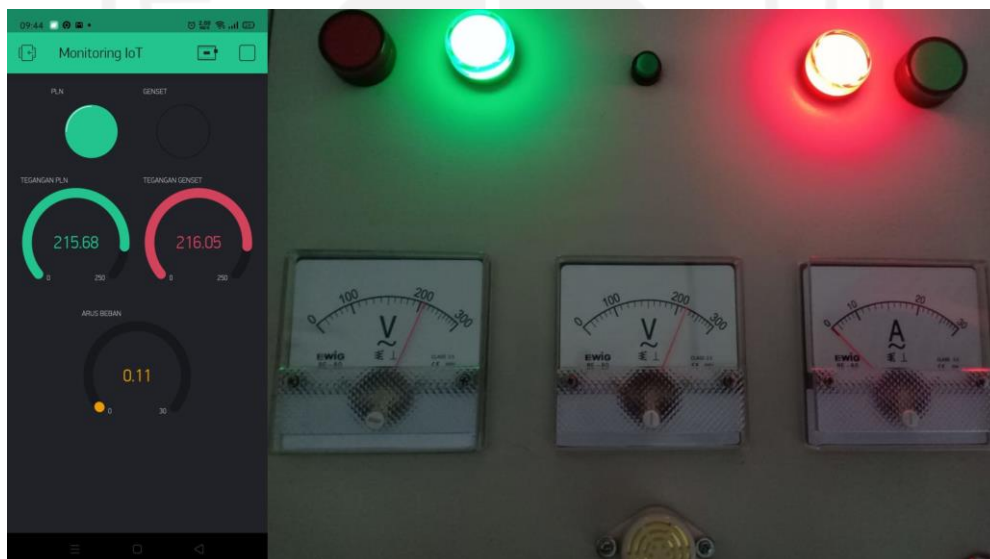
Gambar 5.10 Pengujian sistem telemonitoring IoT dengan kedua sumber listrik aktif
