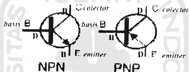
Gambar 2.9 Simbol Transistor NPN dan PNP
