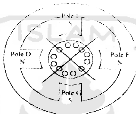
Gambar 2.4 Arah Arus Armatur untuk Putaran Searah Jarum Jam
