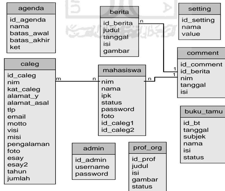
Gambar 4.12 Relasi Tabel
