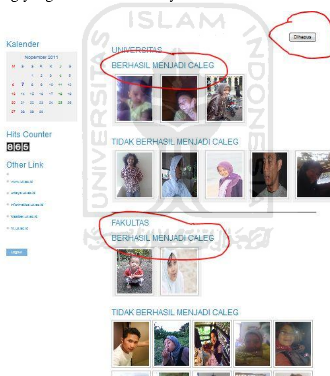
Gambar 5.46 Hasil Seleksi
