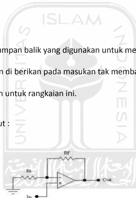
Gambar 3.7. Penguat tak Membalik
