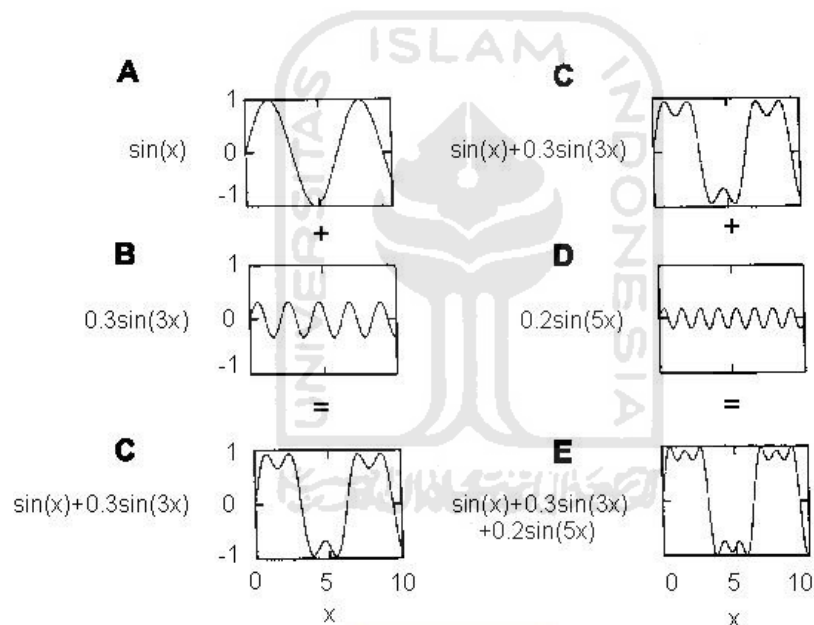
Gambar 3.8 Pembentukan Gelombang
