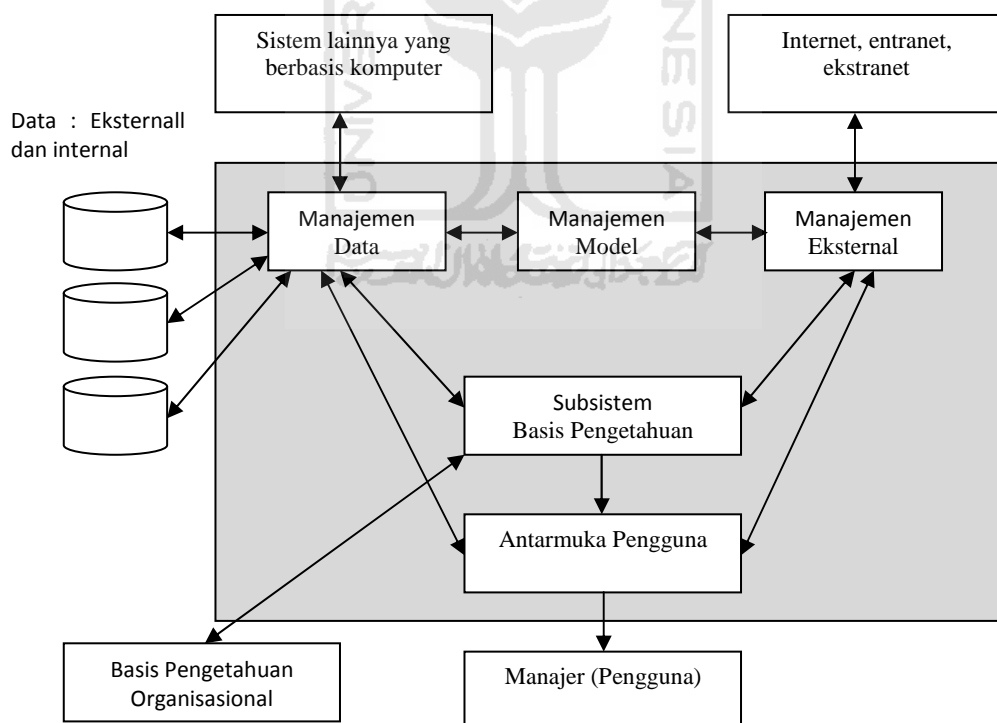
Gambar 2.1 Skematik Sistem Pendukung Keputusan
