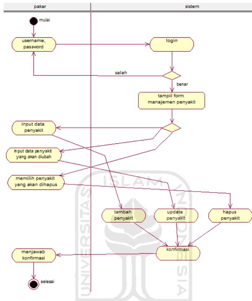
Gambar 4.4 Activity Diagram Manajemen Penyakit
