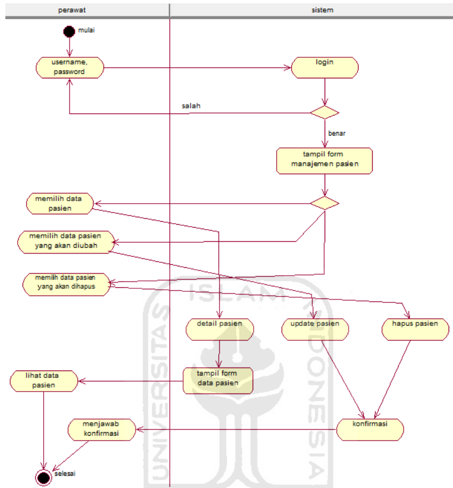
Gambar 4.8 Activity Diagram Manajemen Pasien
