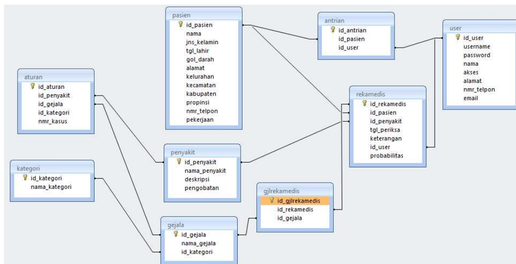
Gambar 4.11 Relasi Antar Table
