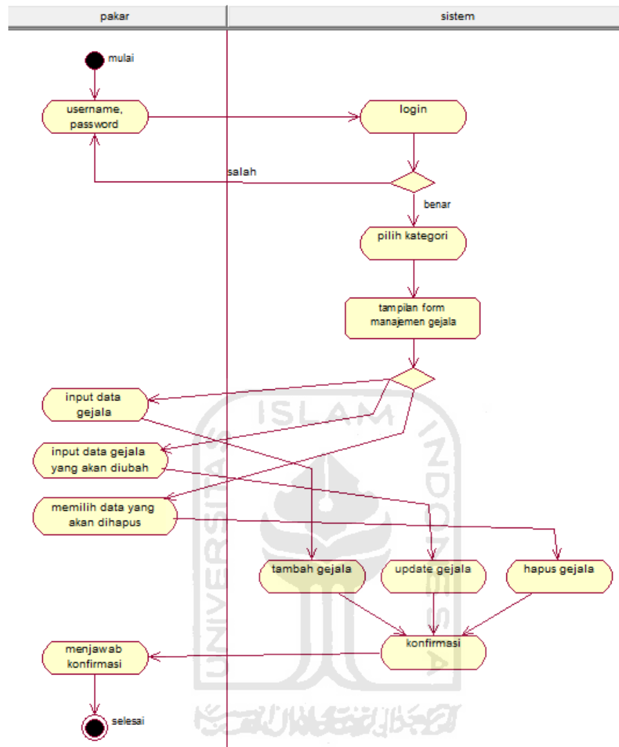
Gambar 4.6 Activity Diagram Manajemen Gejala
