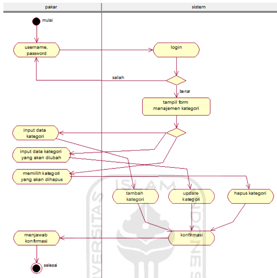
Gambar 4.5 Activity Diagram Manajemen Kategori
