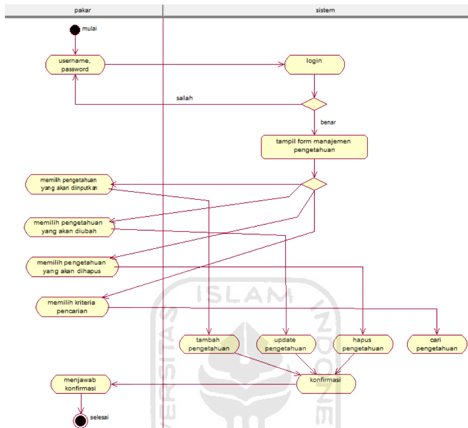
Gambar 4.7 Activity Diagram Manajemen Pengetahuan
