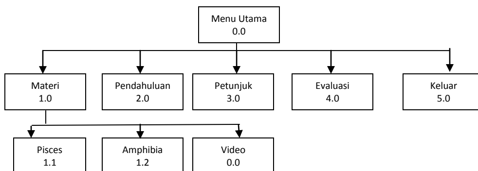
Gambar 3.1 Diagram HIPO
