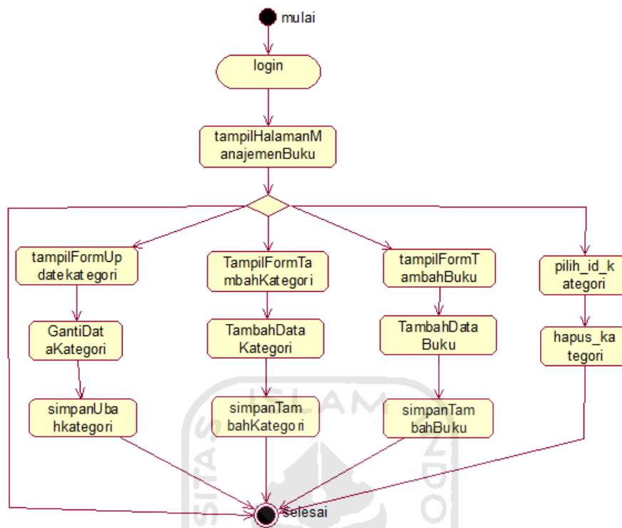
Gambar 4.4. Activity Diagram Manajemen Buku
