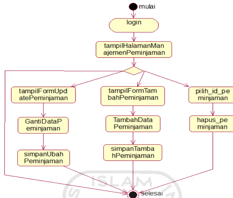
Gambar 4.6. Activity Diagram Manajemen Peminjaman
