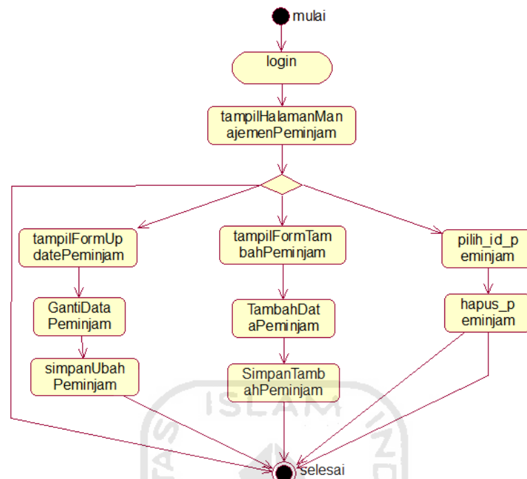
Gambar 4.5. Activity Diagram Manajemen Peminjam
