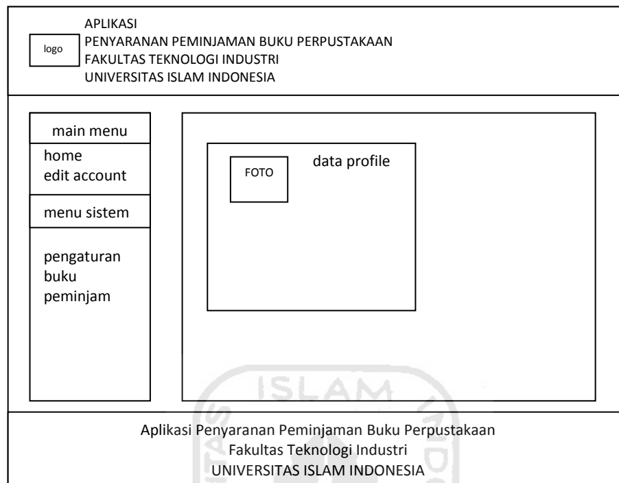
Gambar 4.10. Halaman Home Kaperpus
