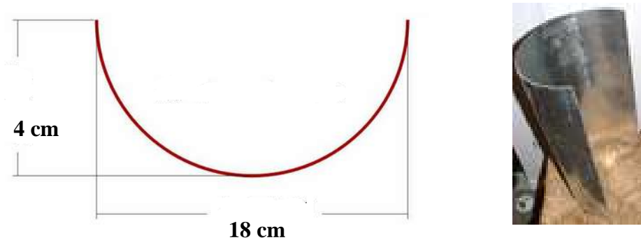
Gambar 3.2. Perancangan sudu
