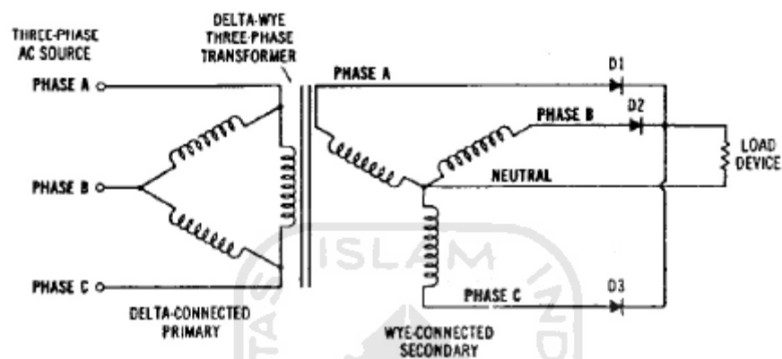
Gambar 2.12. Penyearah setengah gelombang 3 fasa
