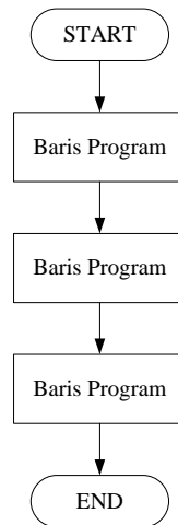
Gambar 2.8 Flowchart Struktur Urut
