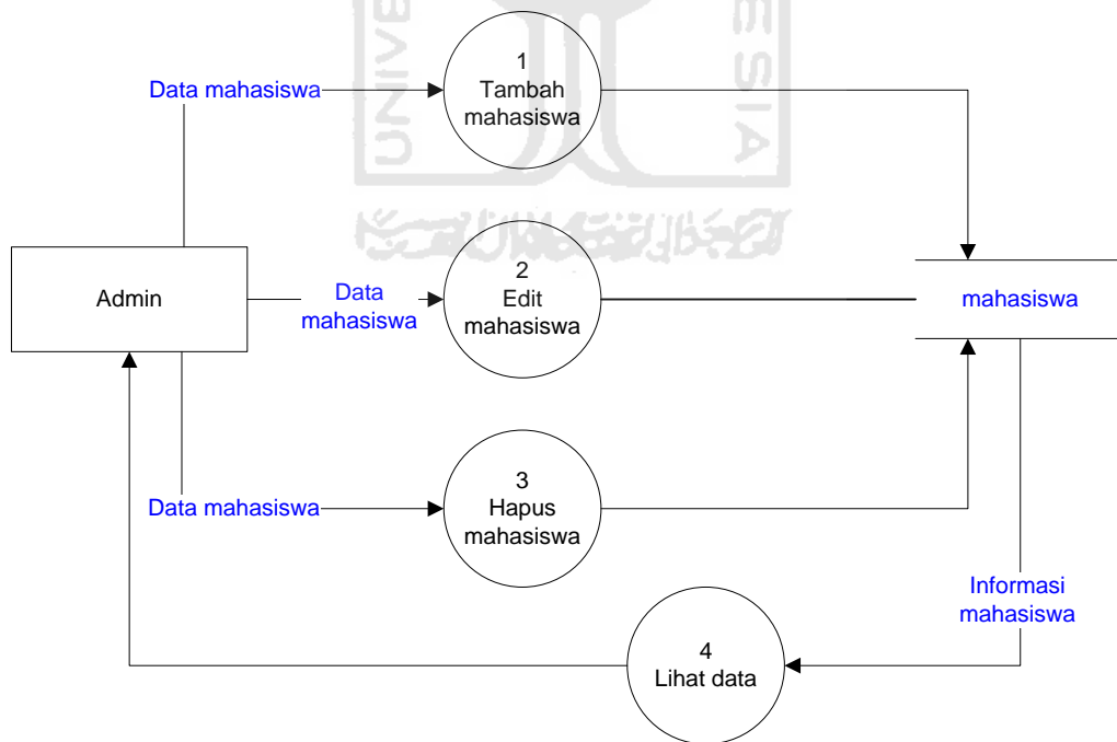
Gambar 4.36 DFD level-2 Mahasiswa
