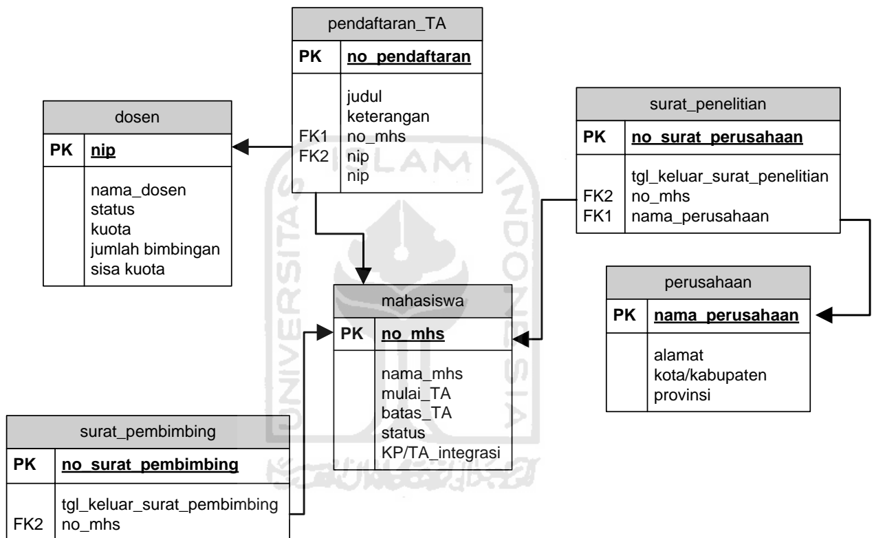
Gambar 4.32 Relasi Antar Tabel
