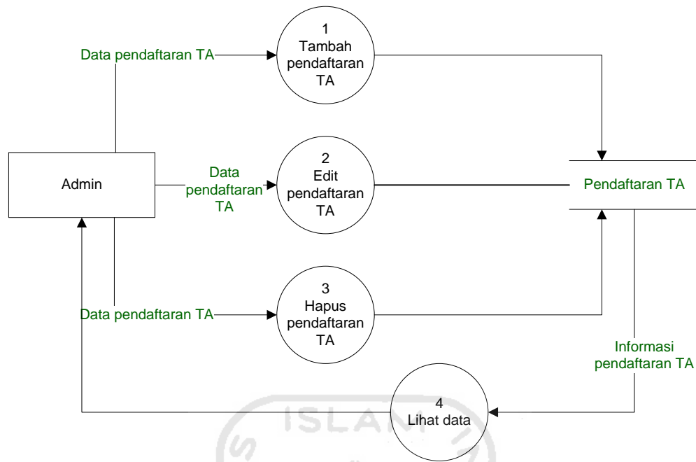
Gambar 4.35 DFD level-2 Pendaftaran TA
