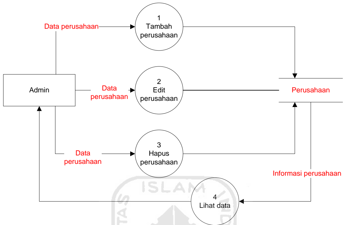
Gambar 4.37 DFD level-2 Perusahaan
