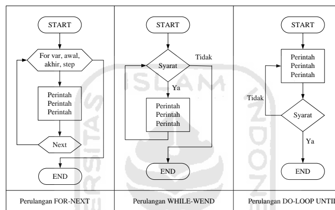
Gambar 2.10 Flowchart Struktur Perulangan
