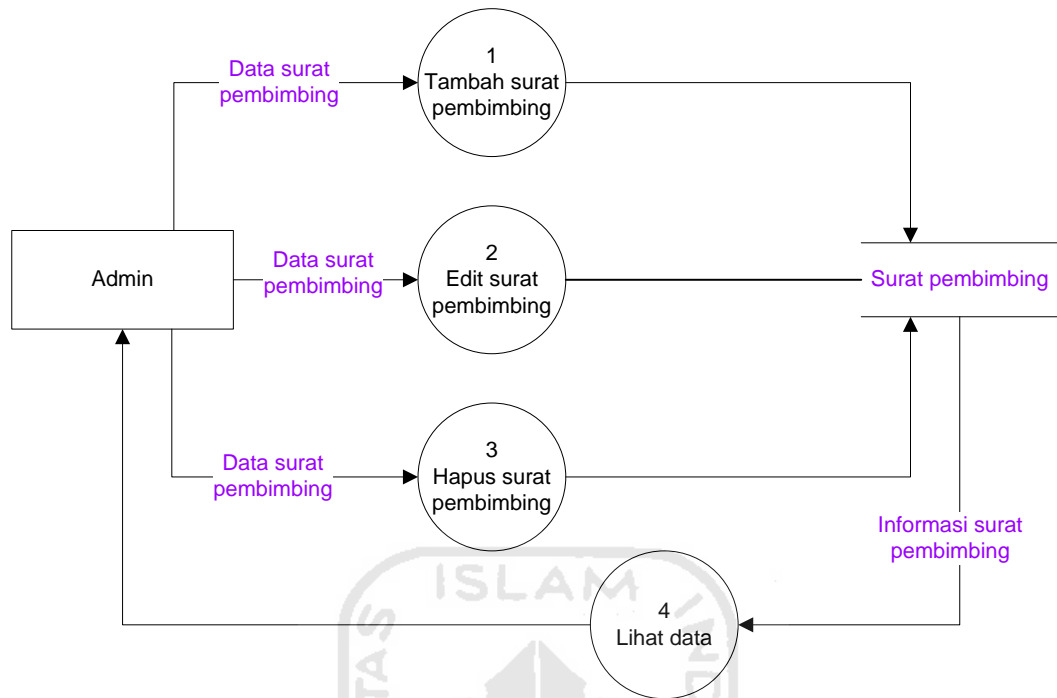
Gambar 4.39 DFD level-2 Surat Pembimbing
