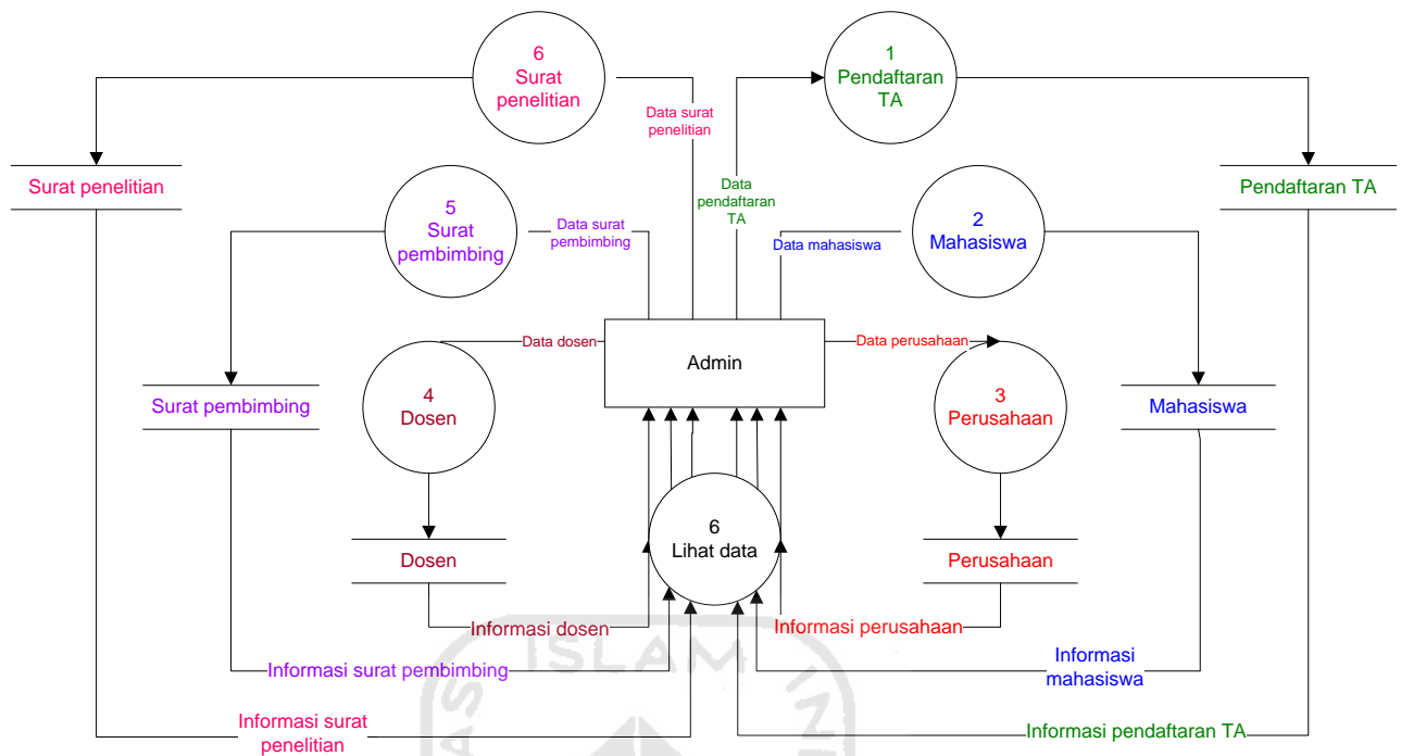
Gambar 4.34 DFD level-1
