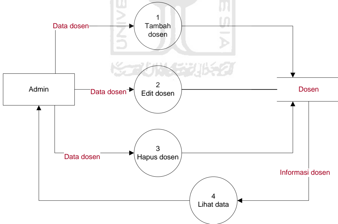
Gambar 4.38 DFD level-2 Dosen
