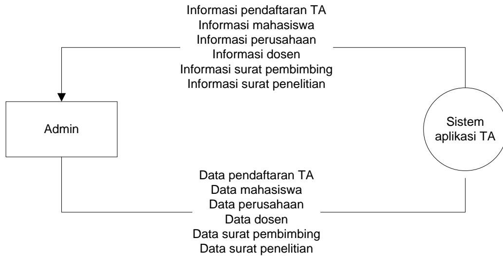
Gambar 4.33 DFD level-0
