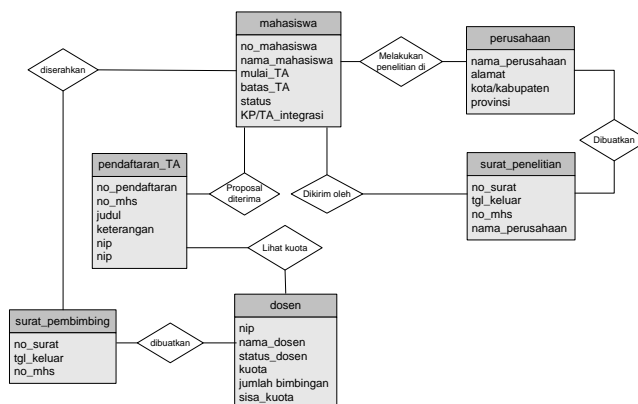
Gambar 4.31 ERD Sistem Aplikasi TA
