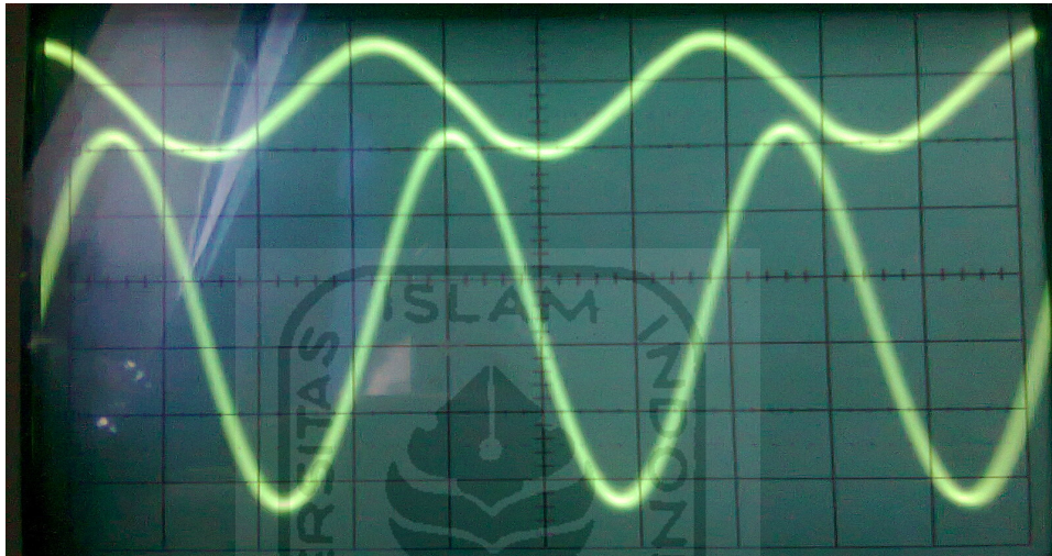
Gambar 4.3 Keluaran Sensor Faraday pada posisi solenoid di atas
