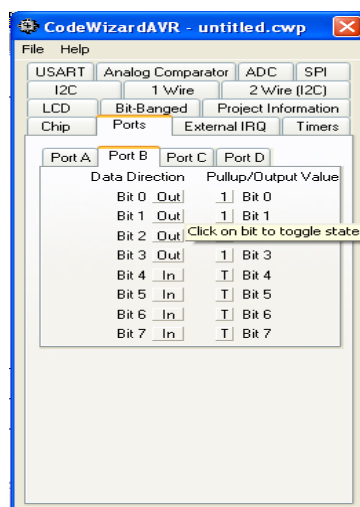
Gambar 3.12 Pengaturan fungsi port mikokontroler pada CodeVision AVR
