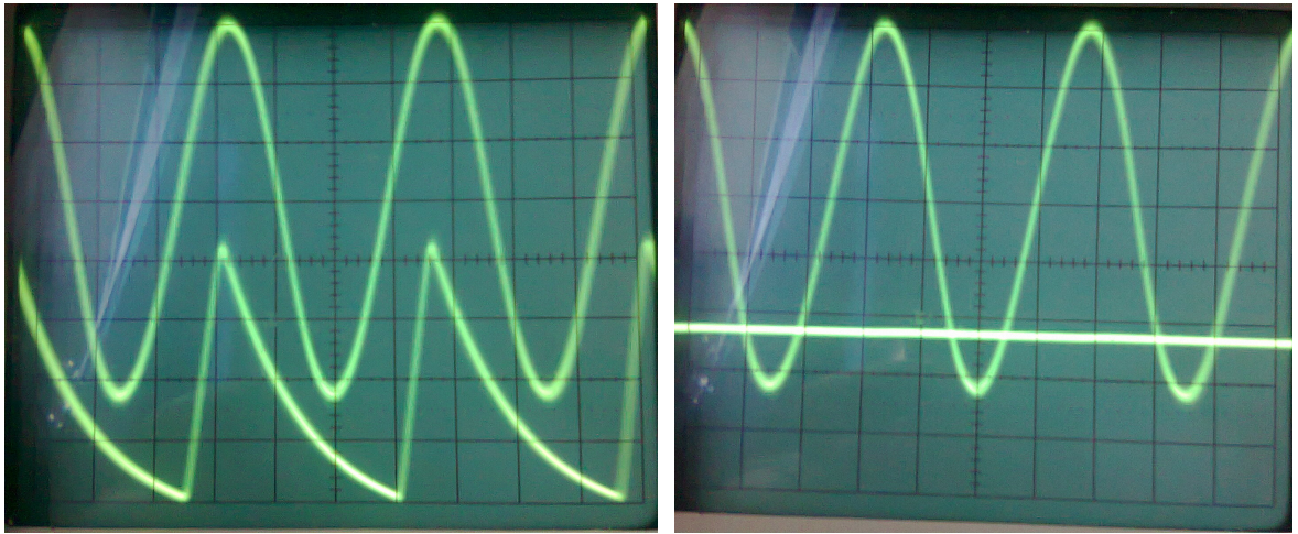
Gambar 4.7 Hasil dari rangkaian penyearah, posisi solenoid di bawah
