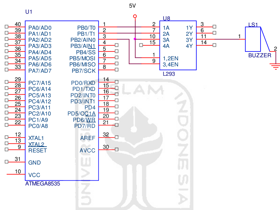
Gambar 3.9 Rangkaian Buzer
