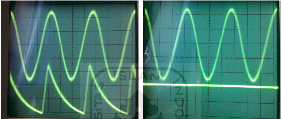
Gambar 4.6 Hasil dari rangkaian penyearah, posisi solenoid di atas
