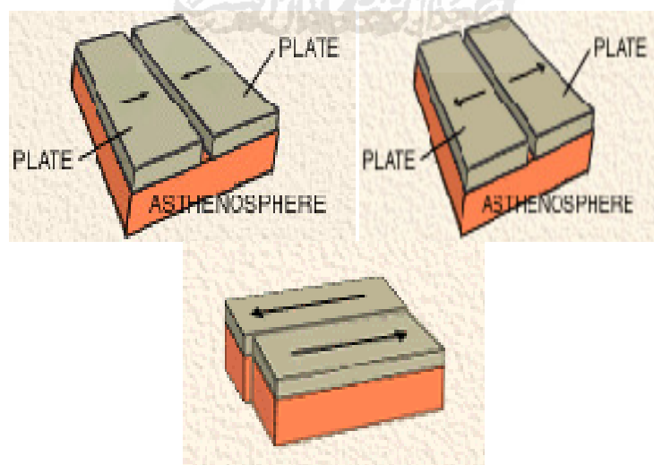
Gambar 2.3 Arah Pergerakan Lempeng Tektonik
