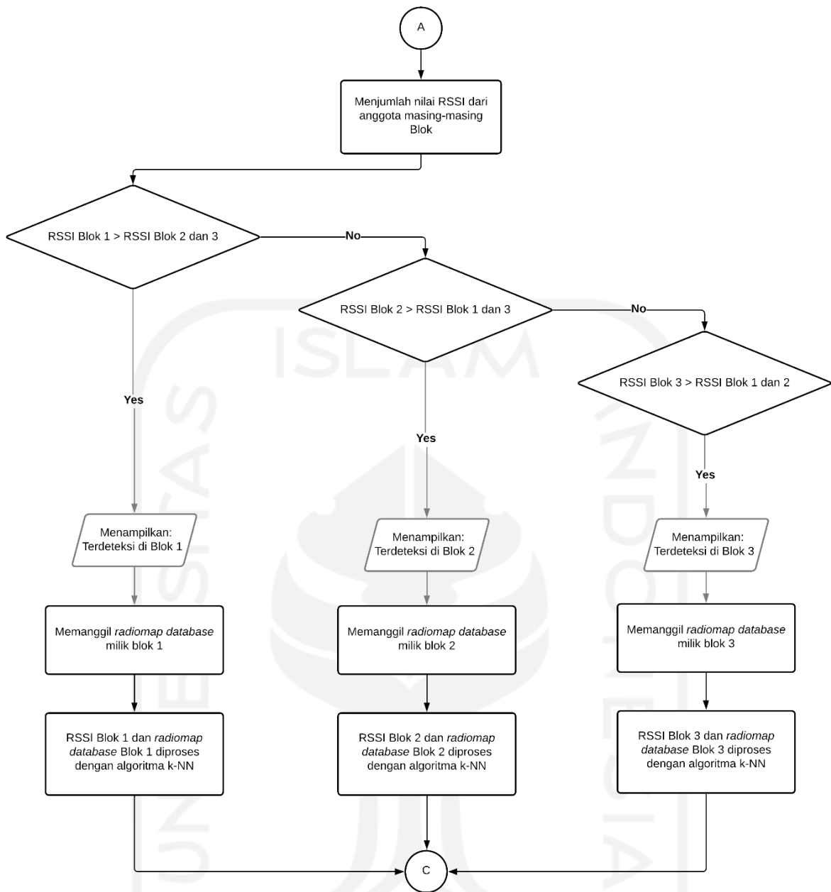
Gambar 4.2. Flow chart sistem bagian penentuan blok lokasi.
