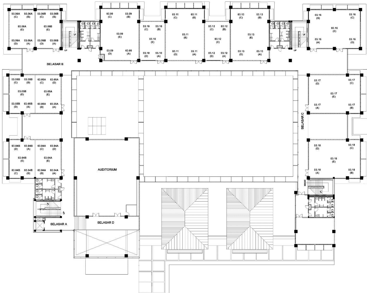
Gambar 4.4. Denah lantai 3 Gedung FTI UII
