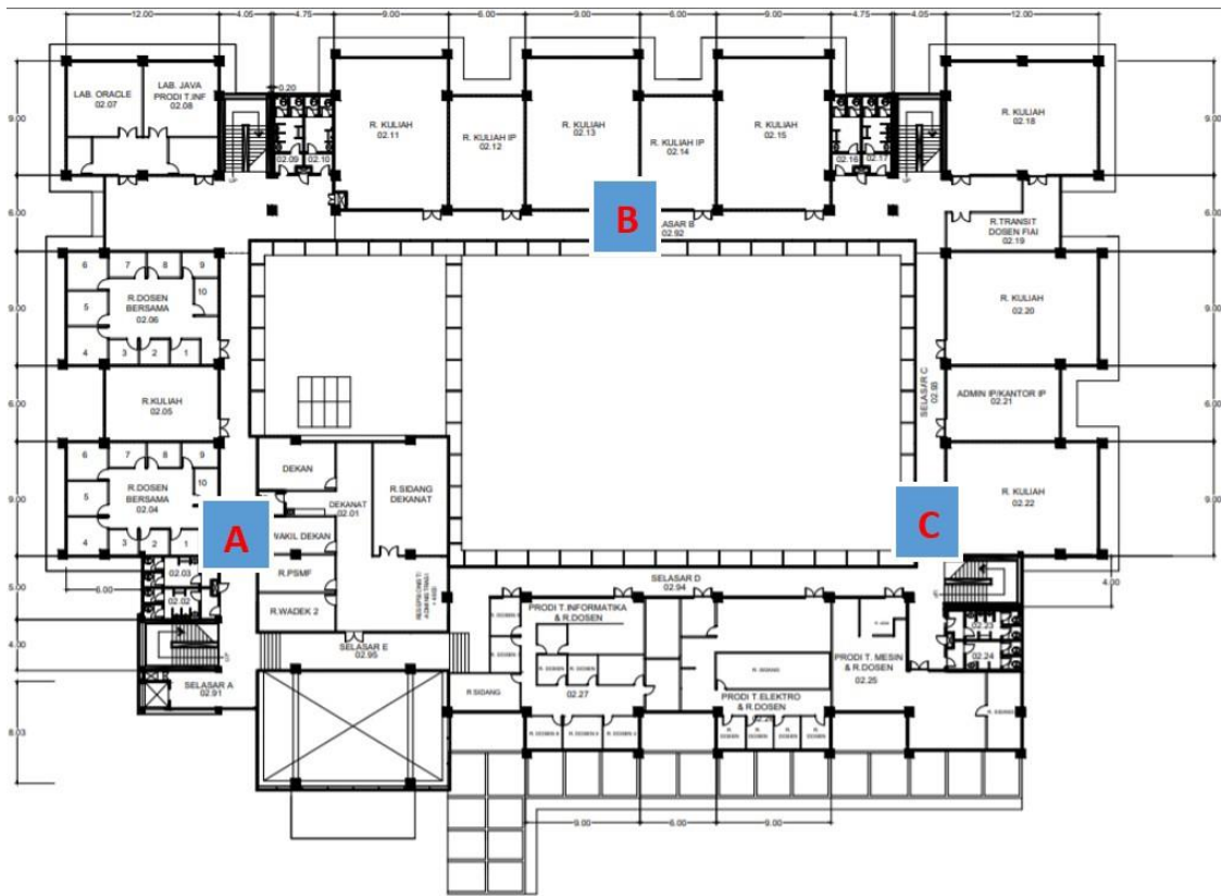
Gambar 3.5. Ilustrasi titik uji scanning sinyal WiFi di lantai 2.
