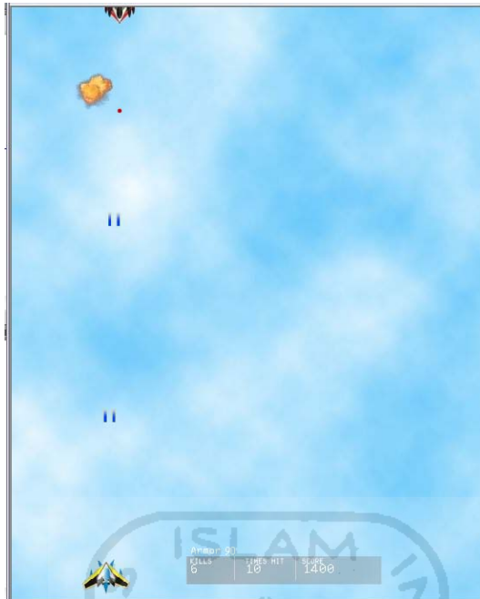
Gambar 4.3 Pesawat Menembak
