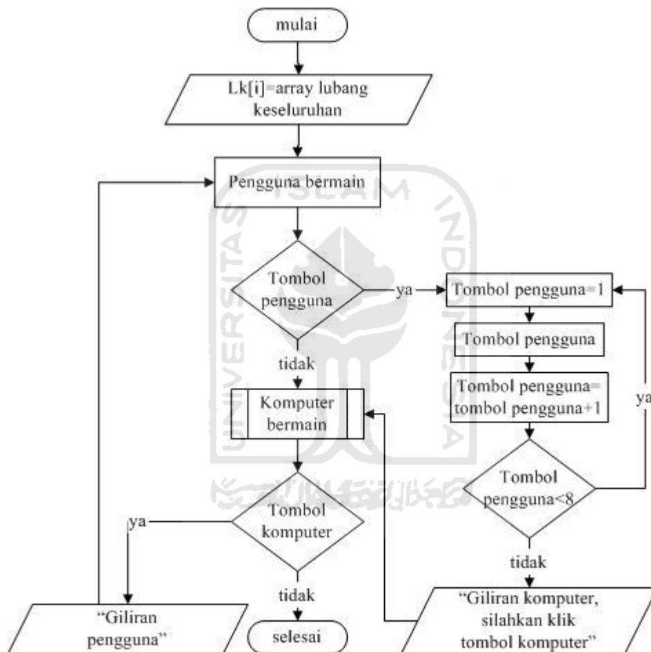
Gambar 4.4 Flowchart Aplikasi Permainan Congklak
