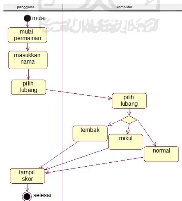
Gambar 4.3 Activity Diagram Memulai Permainan Congklak
