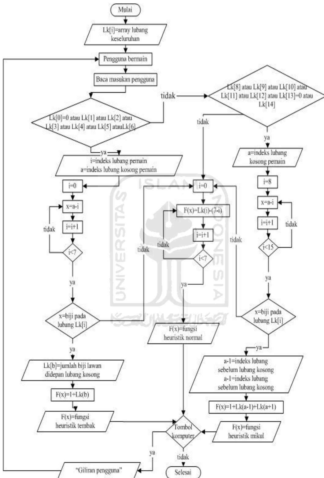
Gambar 4.5 Flowchart Komputer Bermain
