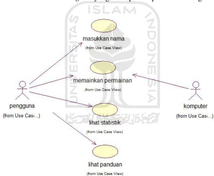
Gambar 4.1 Use Case Diagram Aplikasi Permainan Congklak
