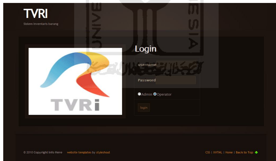
Gambar 4.1 Halaman Login
