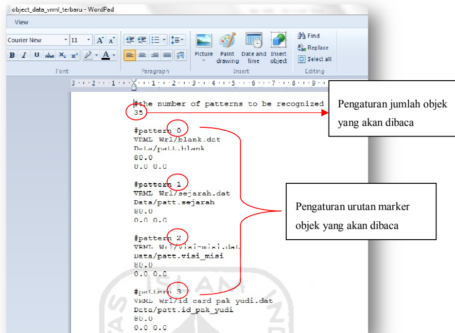
Gambar 3.25 Isi dari data object_data_vrml dan proses pengaturan objek data.
