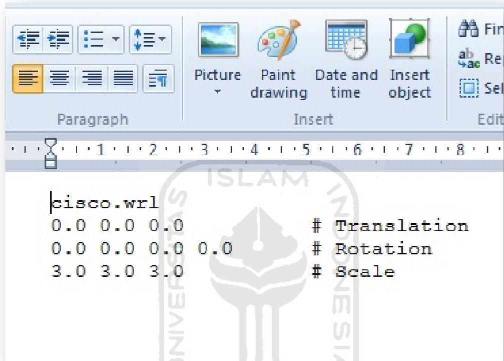
Gambar 3.24 Isi dari file cisco.dat
