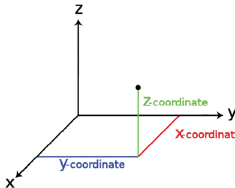
Gambar 2.1 Sistem Koordinat Tiga Dimensi: Sumbu X, Y, Dan Z
