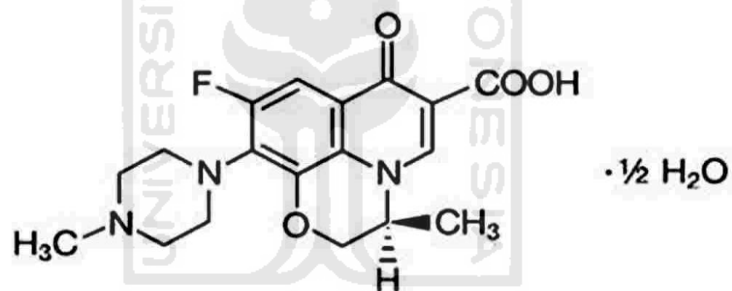
Gambar 1. Struktur Levofloksasin (15) .
