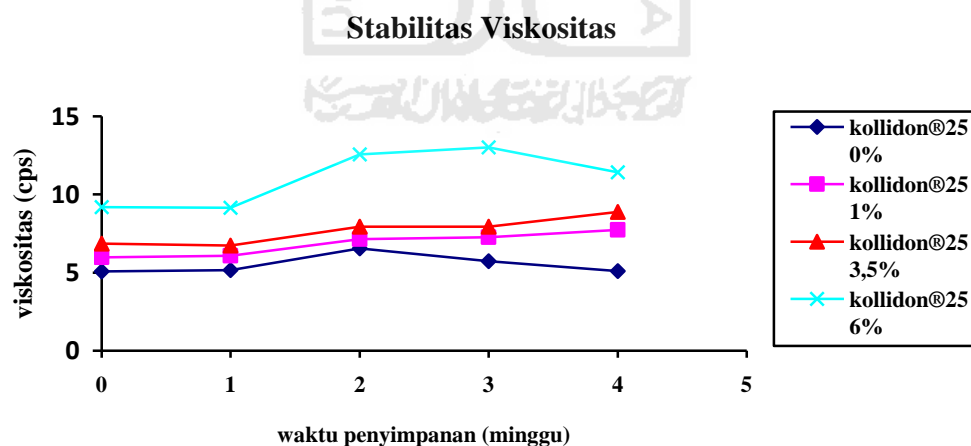
Gambar 11. Grafik hubungan antara viskositas dengan waktu penyimpanan
