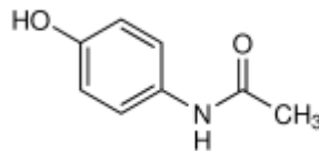
Gambar 1. Rumus struktur parasetamol (10)
