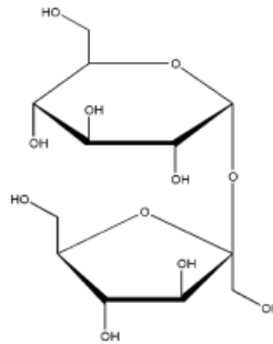
Gambar 5 . Rumus struktur sukrosa (6)
