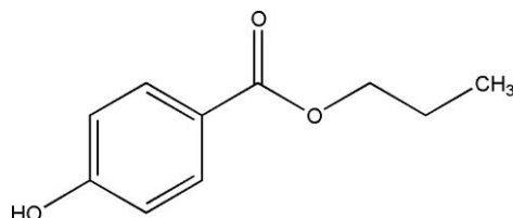
Gambar 7. Rumus struktur propilparaben(6).
