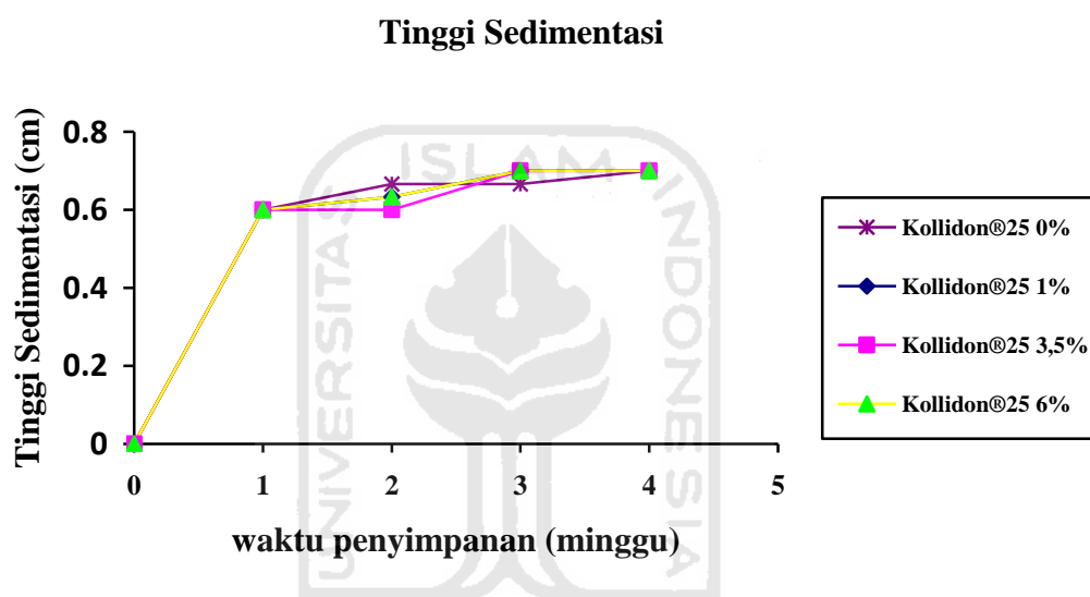
Gambar 9. Grafik hubungan tinggi sedimentasi dengan waktu penyimpanan.
