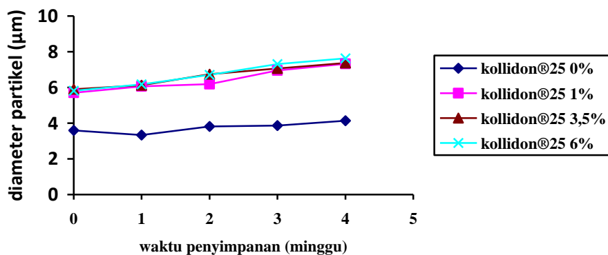
Gambar 12. Grafik hubungan diameter partikel rata-rata dengan waktu penyimpanan.
