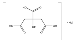
Gambar 3. Rumus struktur asam sitrat.
