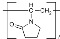
Gambar 2. Struktur kimia Kollidon ® 25 (10)
