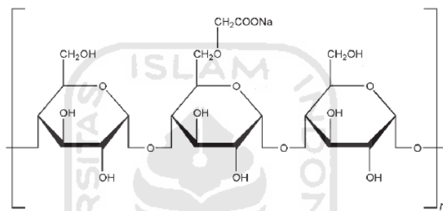
Gambar 5. Struktur Primogel (5) .
