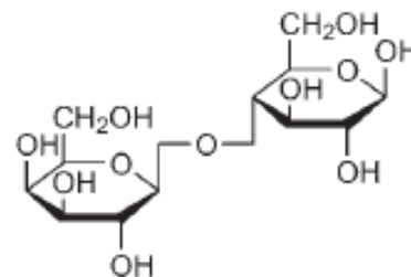
Gambar 4. Struktur Laktosa (5) .
