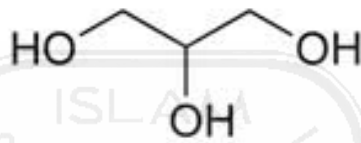
Gambar 6. Struktur Gliserin (39)
