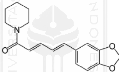
Gambar 2. Struktur Piperin (12).
