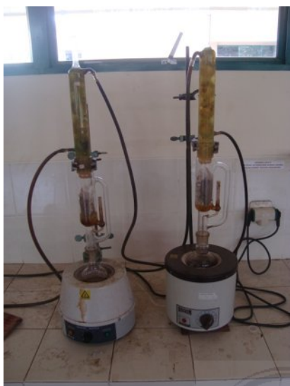
Alat Sokhletasi
