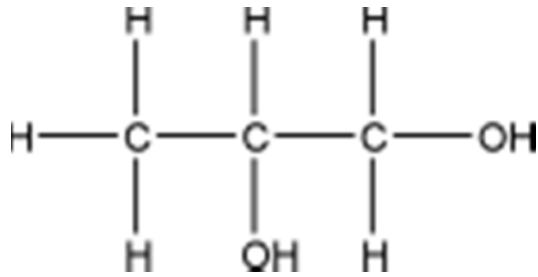
Gambar 5. Struktur Kimia Propilen glikol (24).
