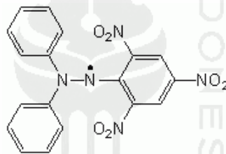
Gambar 4. Struktur DPPH ( 1,1-Diphenyl-2-picrylhydrazyl )
