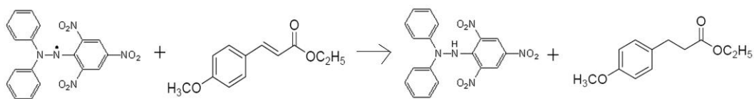
Gambar 12. Mekanisme Reaksi DPPH dan Etil Para Metoksi Sinamat
