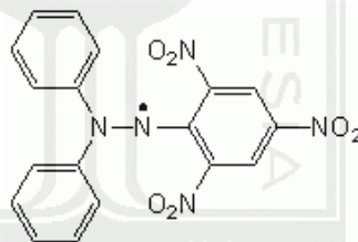
Gambar 3. Struktur DPPH (1,1 Diphenyl-2-picrylhidrazyl)
