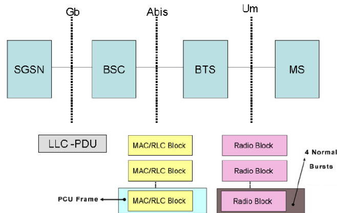
Gambar 2.10 Aliran data dari SGSN ke MS
