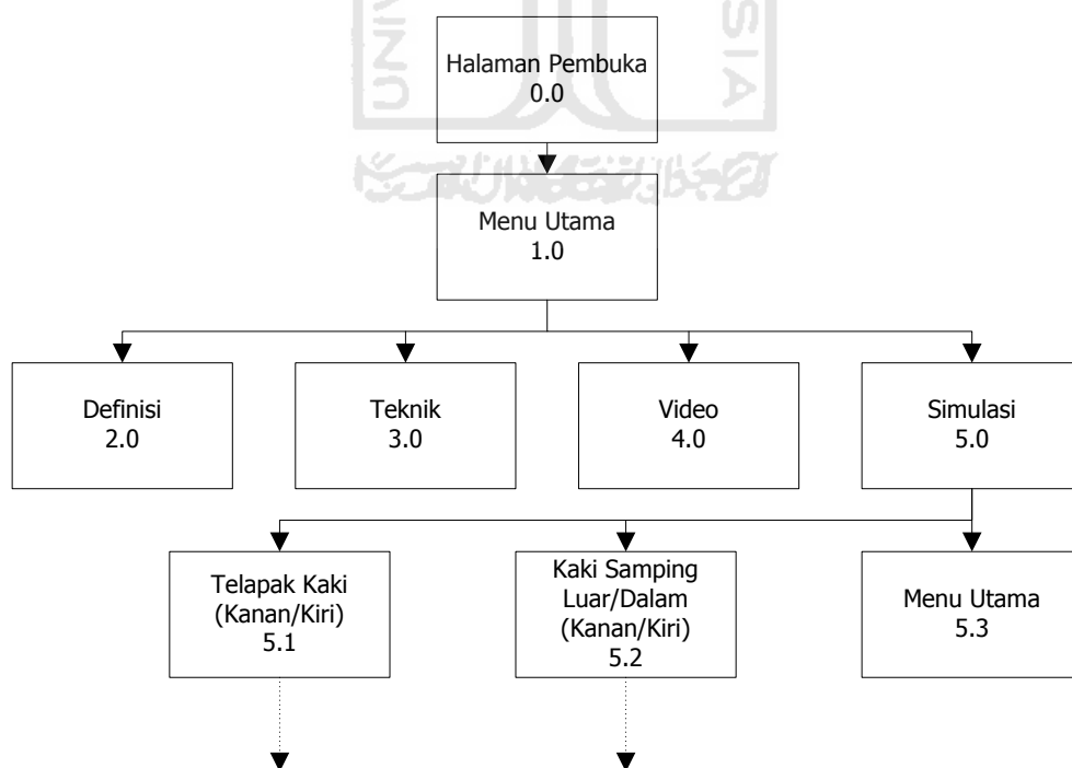
Gambar 3.1.1 Diagram HIPO
