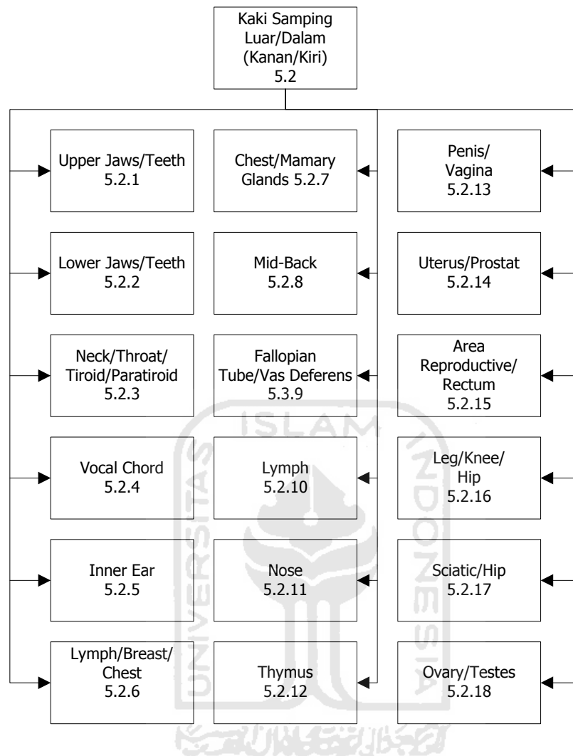
Gambar 3.1.3 Diagram HIPO
