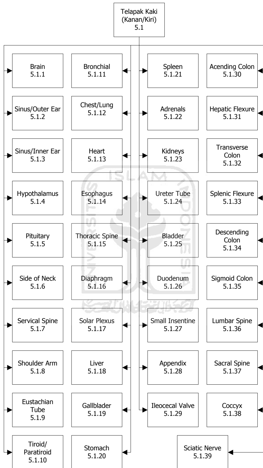
Gambar 3.1.2 Diagram HIPO
