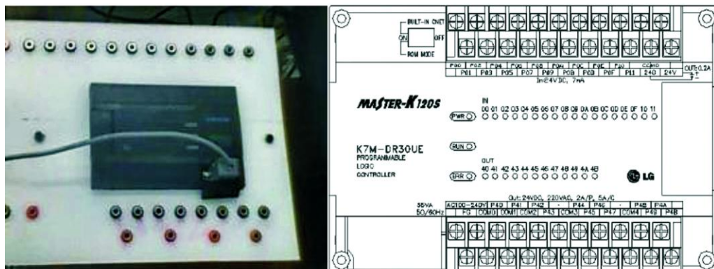
Gambar 2-6 Bentuk fisik PLC master K120S(E) (Sumber data sheet PLC)
