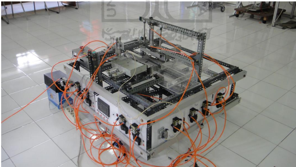
Gambar 4-1 Mesin pengemas pasta gigi jadi
