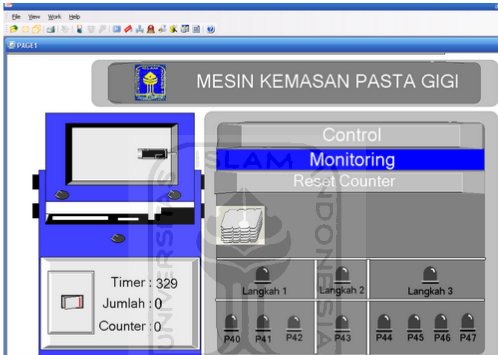
Gambar 4-3 Monitoring dengan CimonD SCADA
