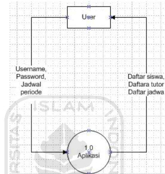
Gambar 3.1 Diagram Konteks
