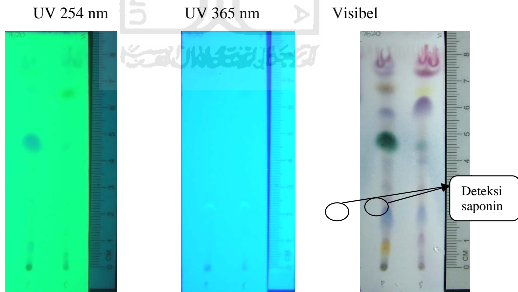
Gambar 14. Hasil uji KLT saponin, dengan fase diam silika gel 60 F 254 dan fase gerak kloroform : metanol dengan perbandingan 95% : 5%.
