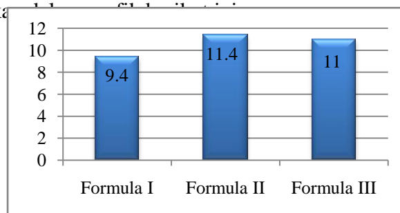
Gambar17. Pengaruh variasi bahan lubrikan terhadap indeks pengetapan massa granul.
