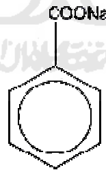
Gambar 10. Struktur Na benzoat (30) .
