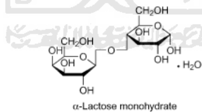
Gambar 9. Struktur laktosa (9) .
