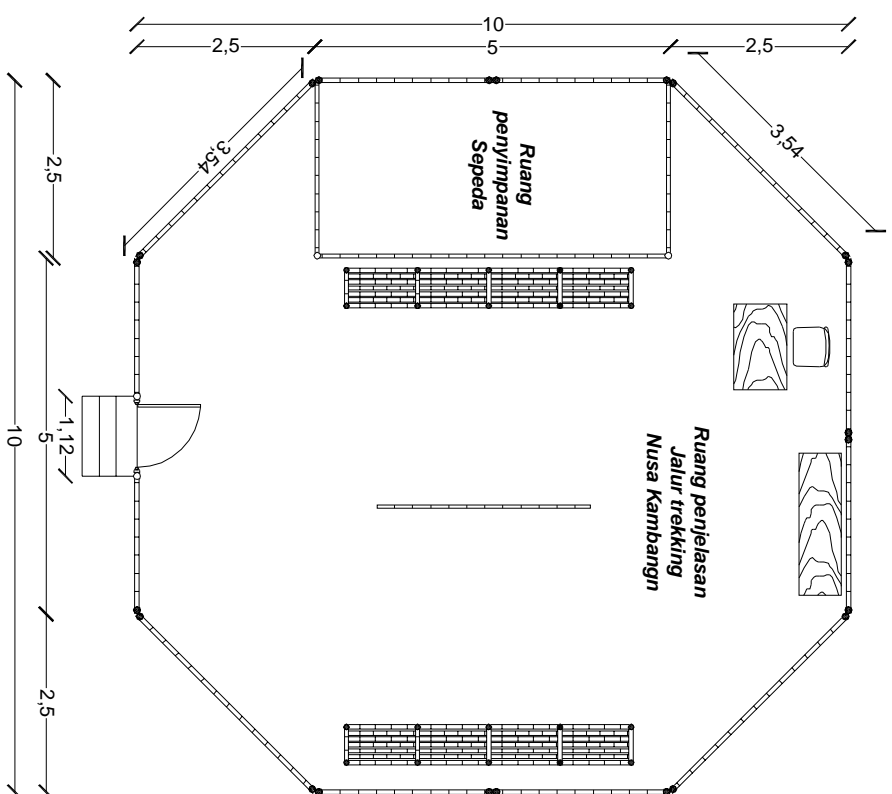
Denah SKALA 1 : 100
