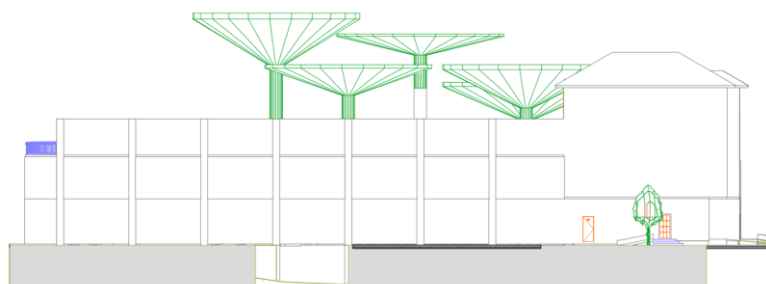
Gambar 4.8 Tampak Selatan
