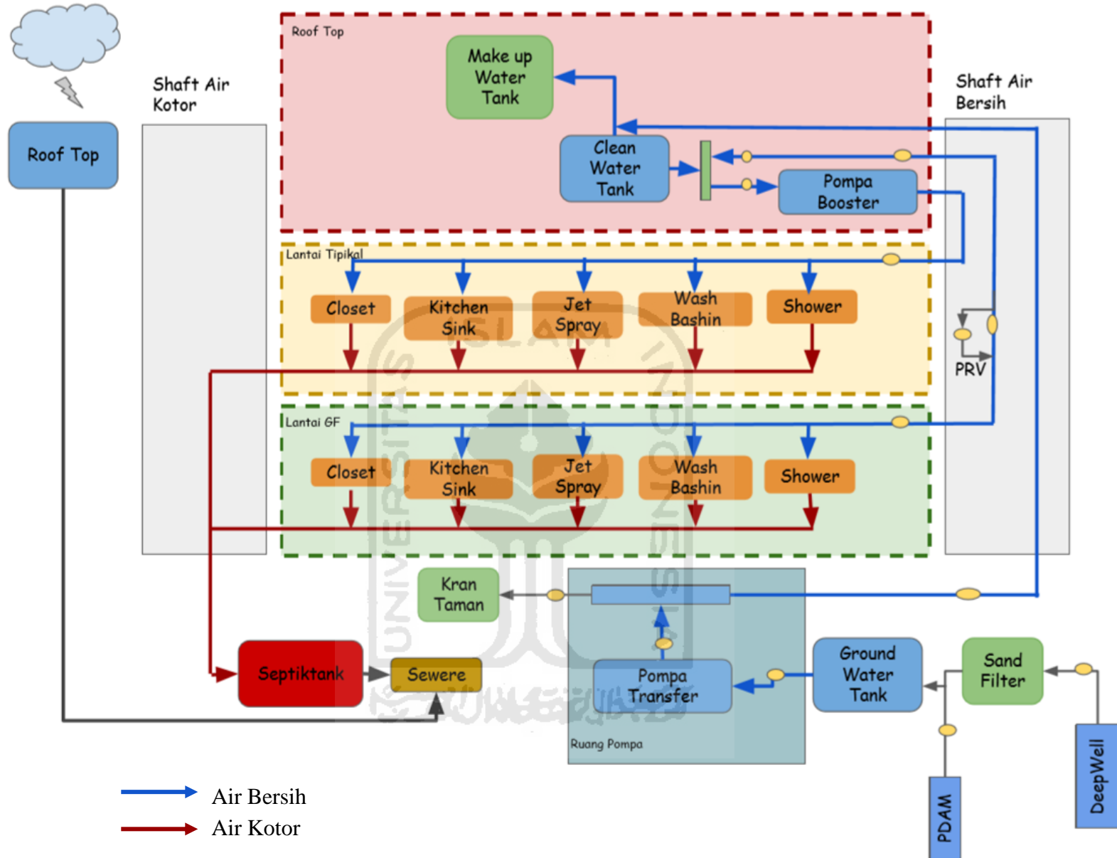
Gambar 3.8 Distribusi Air Bersih
