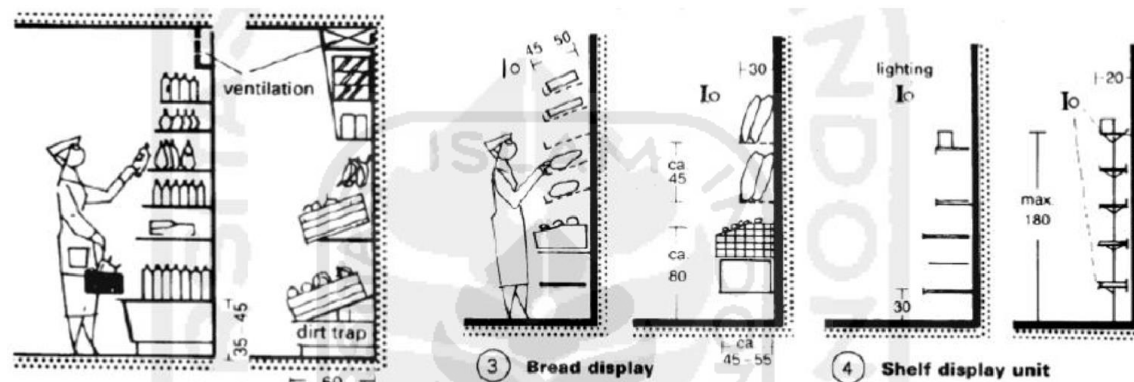
Gambar 3.3 Standar Ukuran Kios
