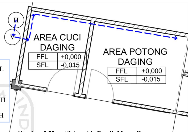
Gambar 5.22 Sistem Air Bersih Massa Dua
