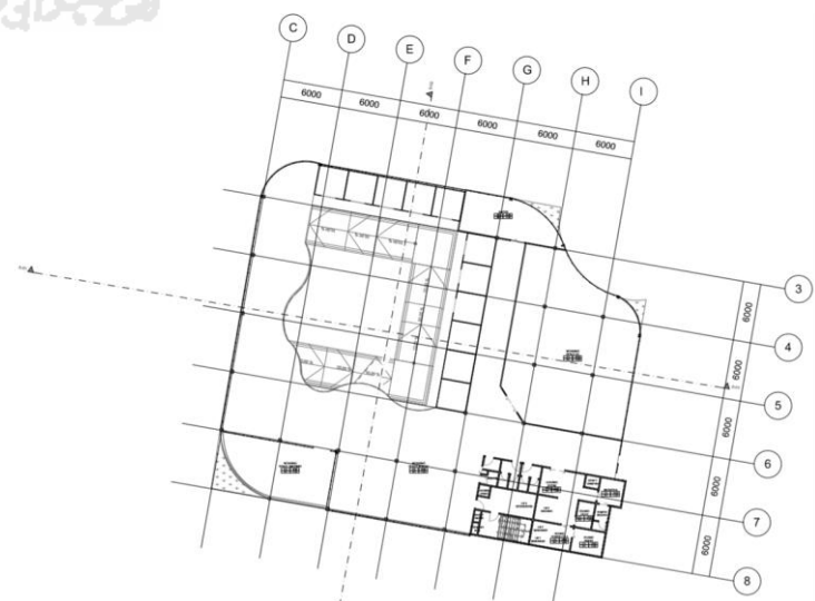
Gambar 5.4 Denah Utama Lantai 3
