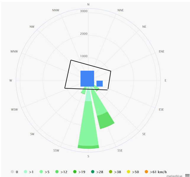
Gambar 3.2 Orientasi terhadap Angin
