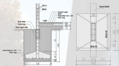
DETAIL PONDASI
