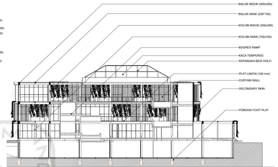
Gambar 5.18 Potongan B-B' Massa Utama
