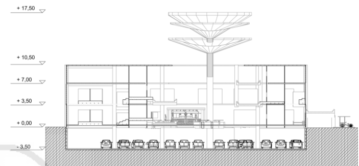
Gambar 4.12 Potongan B-B'
