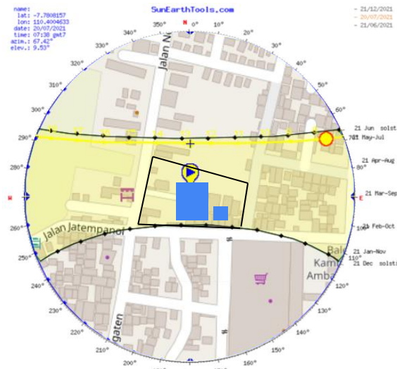
Gambar 3.1 Orientasi terhadap Matahari
