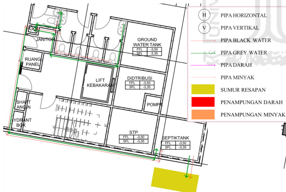
Gambar 5.23 Sistem Air Kotor Massa Utama
