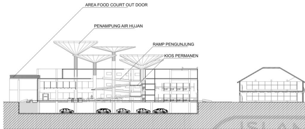
Gambar 4.11 Potongan A-A'
