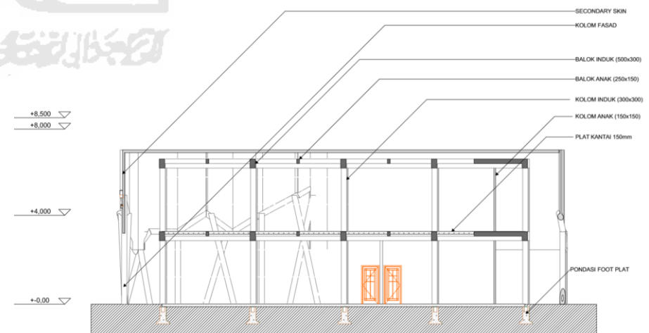
Gambar 5.20 Potongan B-B' Massa Dua
