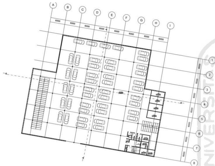
Gambar 5.1 Denah Utama Basement
