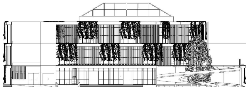
Gambar 5.8 Tampak Timur Massa Utama
