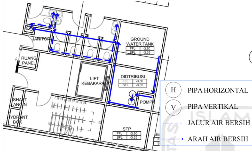
Gambar 5.21 Sistem Air Bersih Massa Utama
