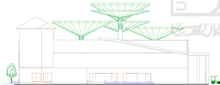
Gambar 4.6 Tampak Timur
