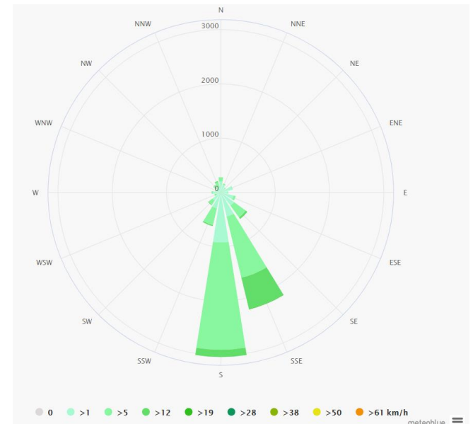
Gambar 2.5 Analisis Angin Kabupaten Sleman Sumber: Meteoblue.com
