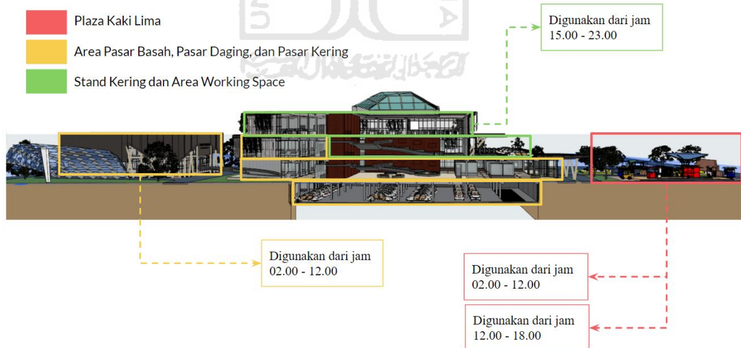
Gambar 3.12 Penyelesaian Change of Time
