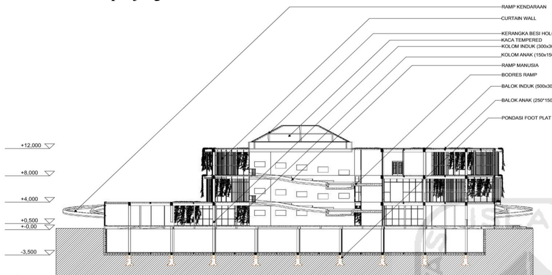
Gambar 5.17 Potongan A-A' Massa Utama
