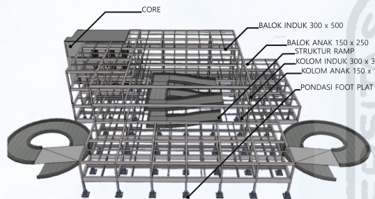
AKSONOMETRI STRUKTUR
