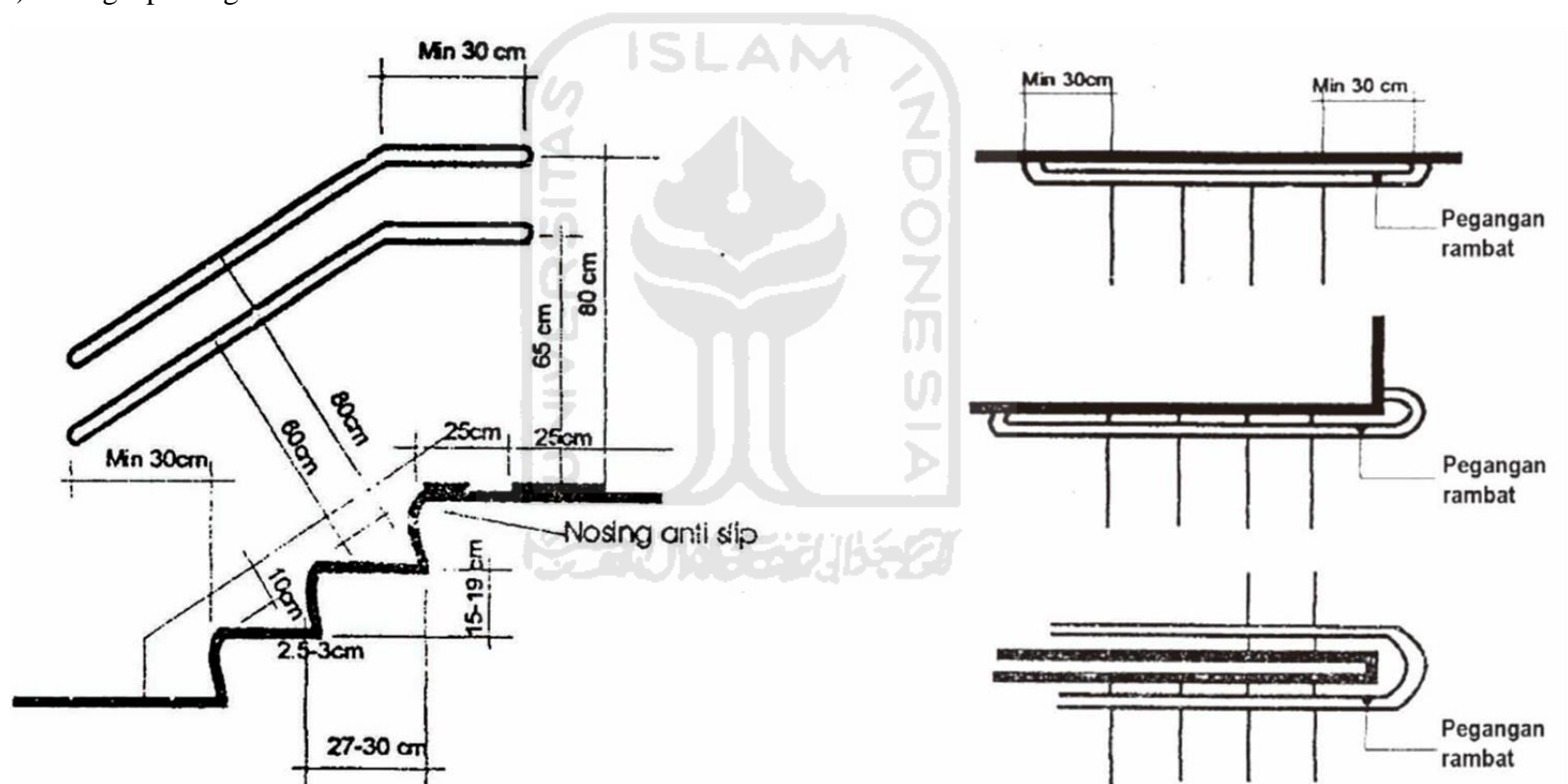
Gambar 3.11 Tangga Darurat
