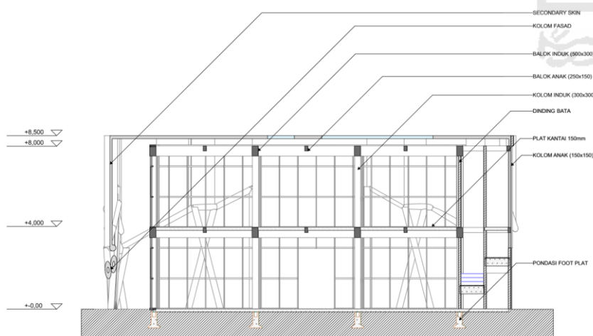
Gambar 5.19 Potongan A-A' Massa Dua
