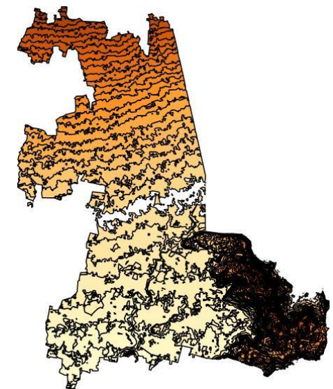
Gambar 2.4 Topografi Kabupaten Sleman
