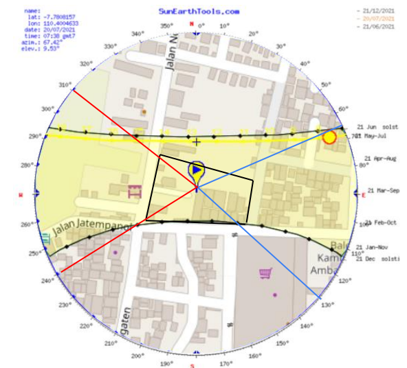
Gambar 2.6 Analisis Matahari Kabupaten Sleman Sumber : sunearthtools.com
