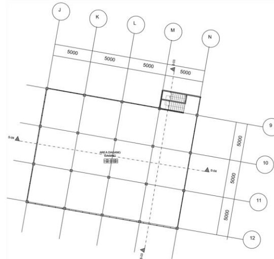
Gambar 5.6 Denah Massa Dua Lantai 2
