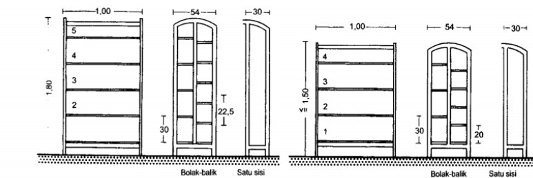
⑭ Rak buku untuk orang dewasa terdiri atas 5 sampai 6 tingkat, sedangkan untuk anak-anak 4 sampai 5 tingkat → ⑫
