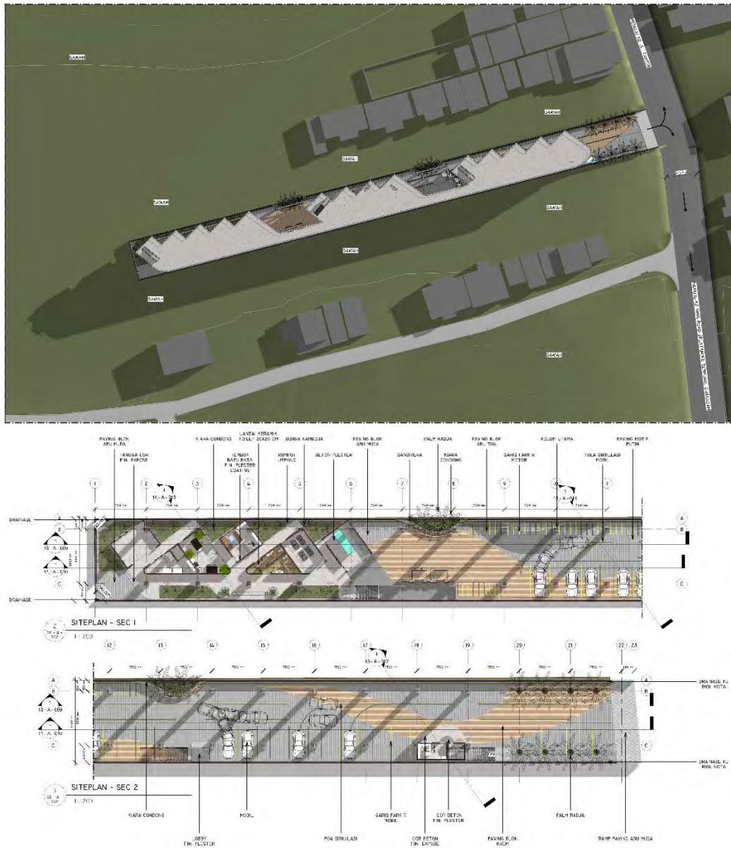
Gambar 52. Kawasan/Siteplan
