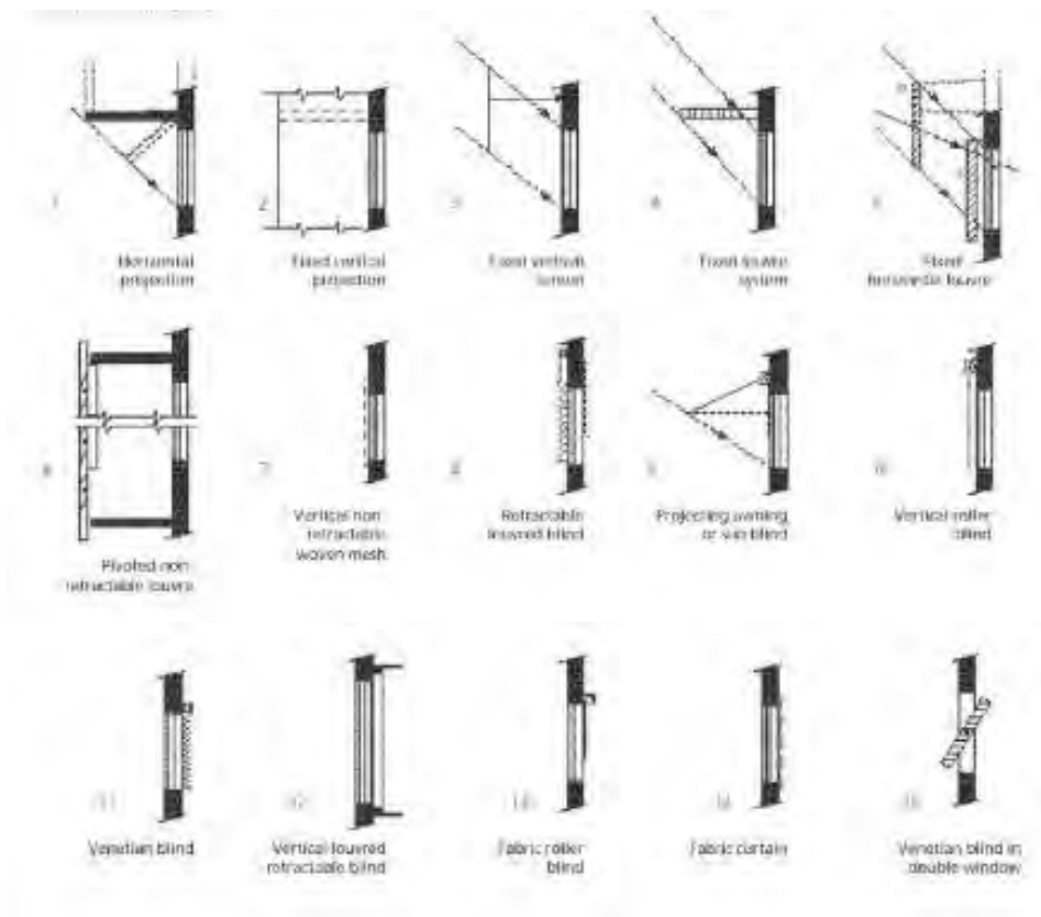
Gambar 2. 31 Shading Eksternal(1-10) dan Shading Internal(11-15) pada bukaan (Sumber: Lighting Guide, LG 10,1999 dalam Manurung, 2012)
