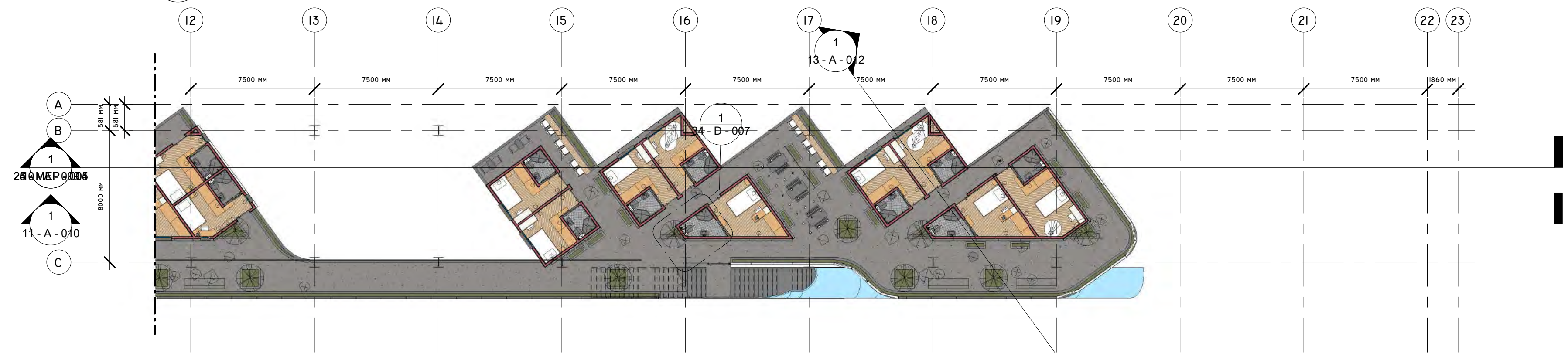
2 07 - A - 006 LEVEL 3 - SEC 2 1 : 200
