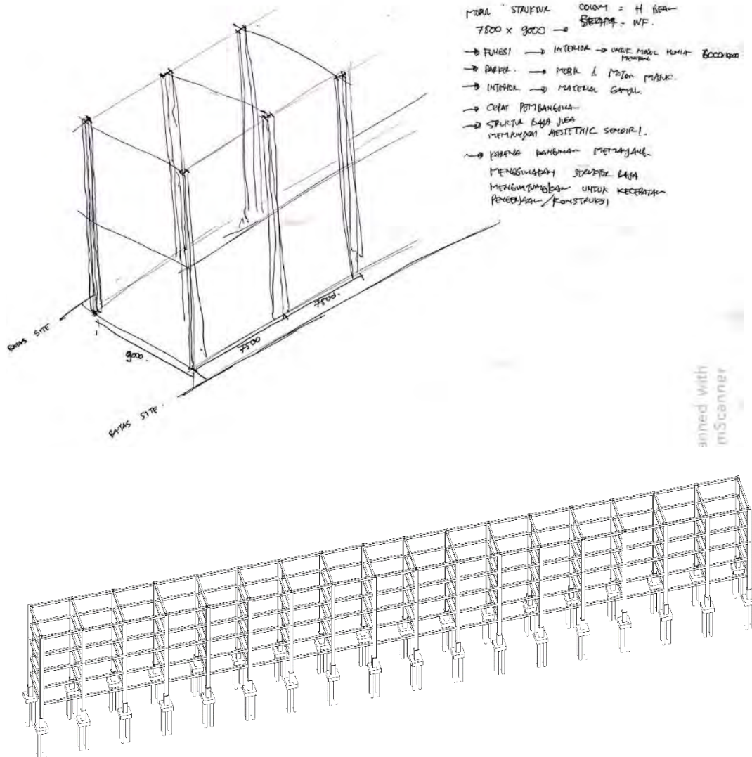
Gambar 47. Skema Struktur
