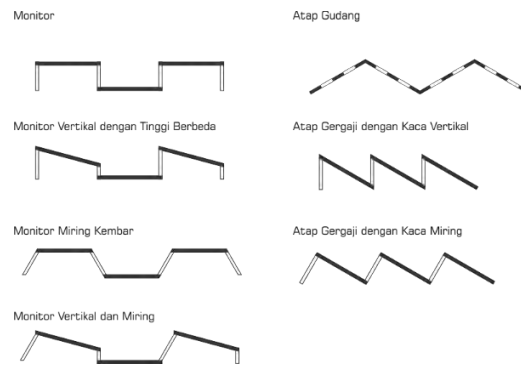
Gambar 2. 27 Jenis pencahayaan yang mengikuti bentuk atap (Sumber: Manurung, 2012)
