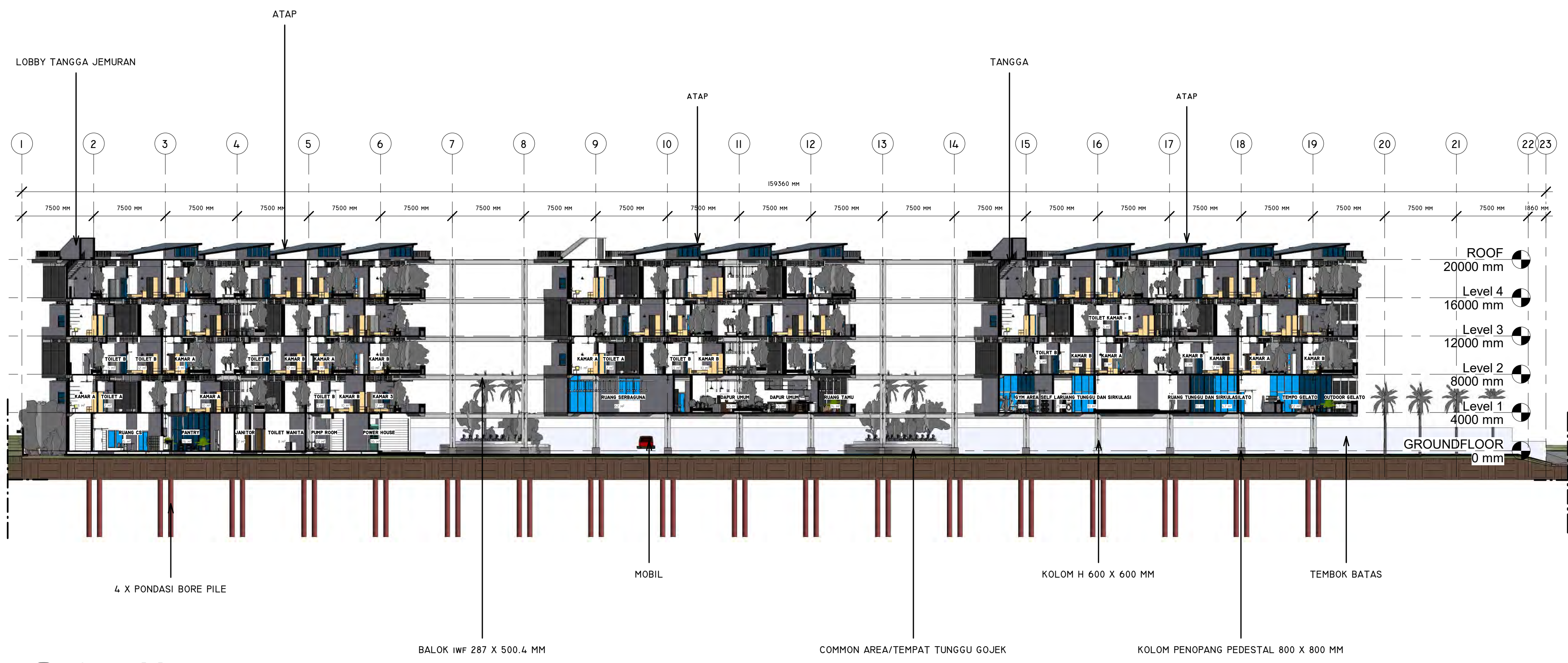
SECTION B-B 1 : 300
