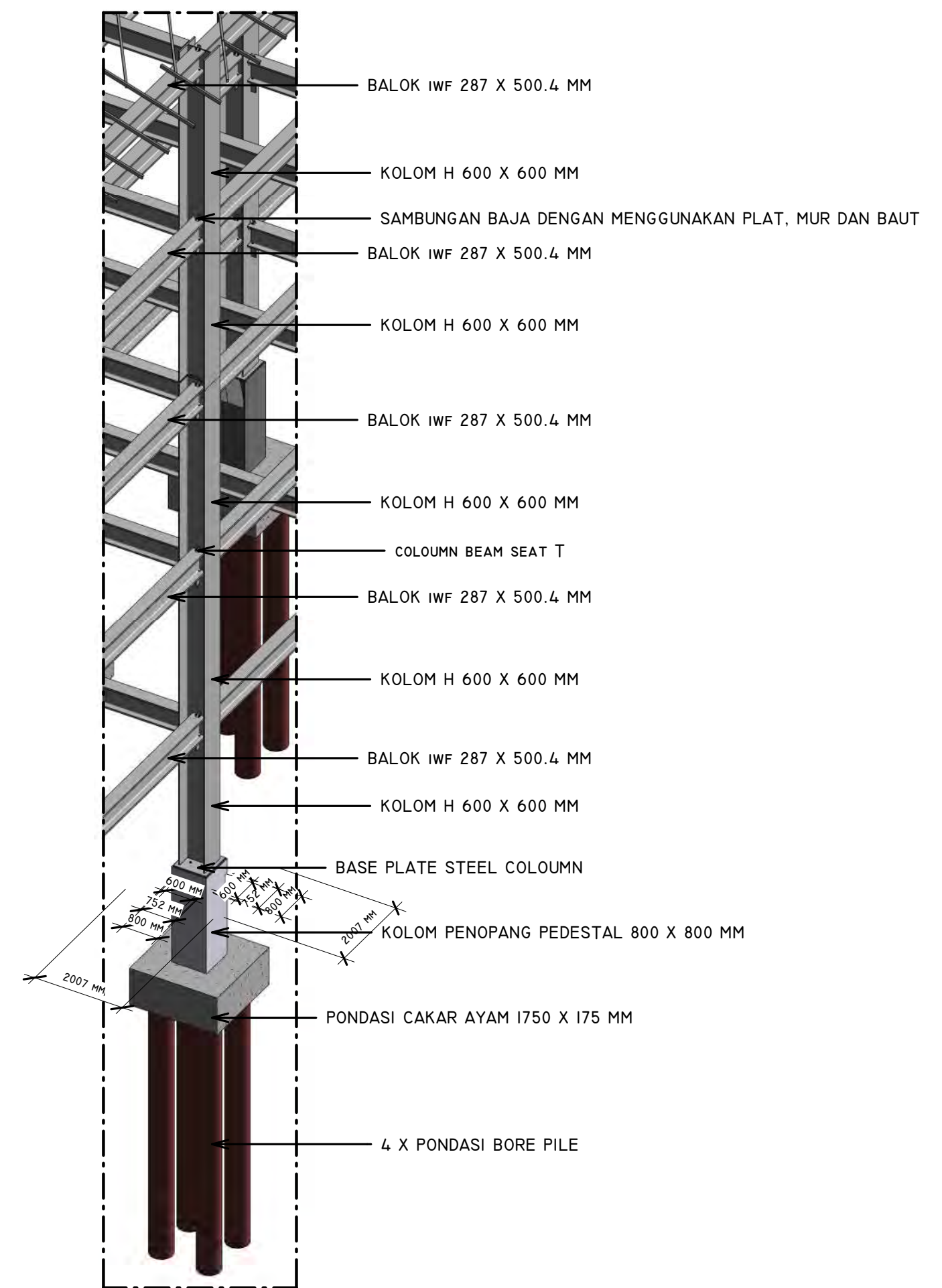
2 20 - S - 001 DETAIL STRUKTUR
