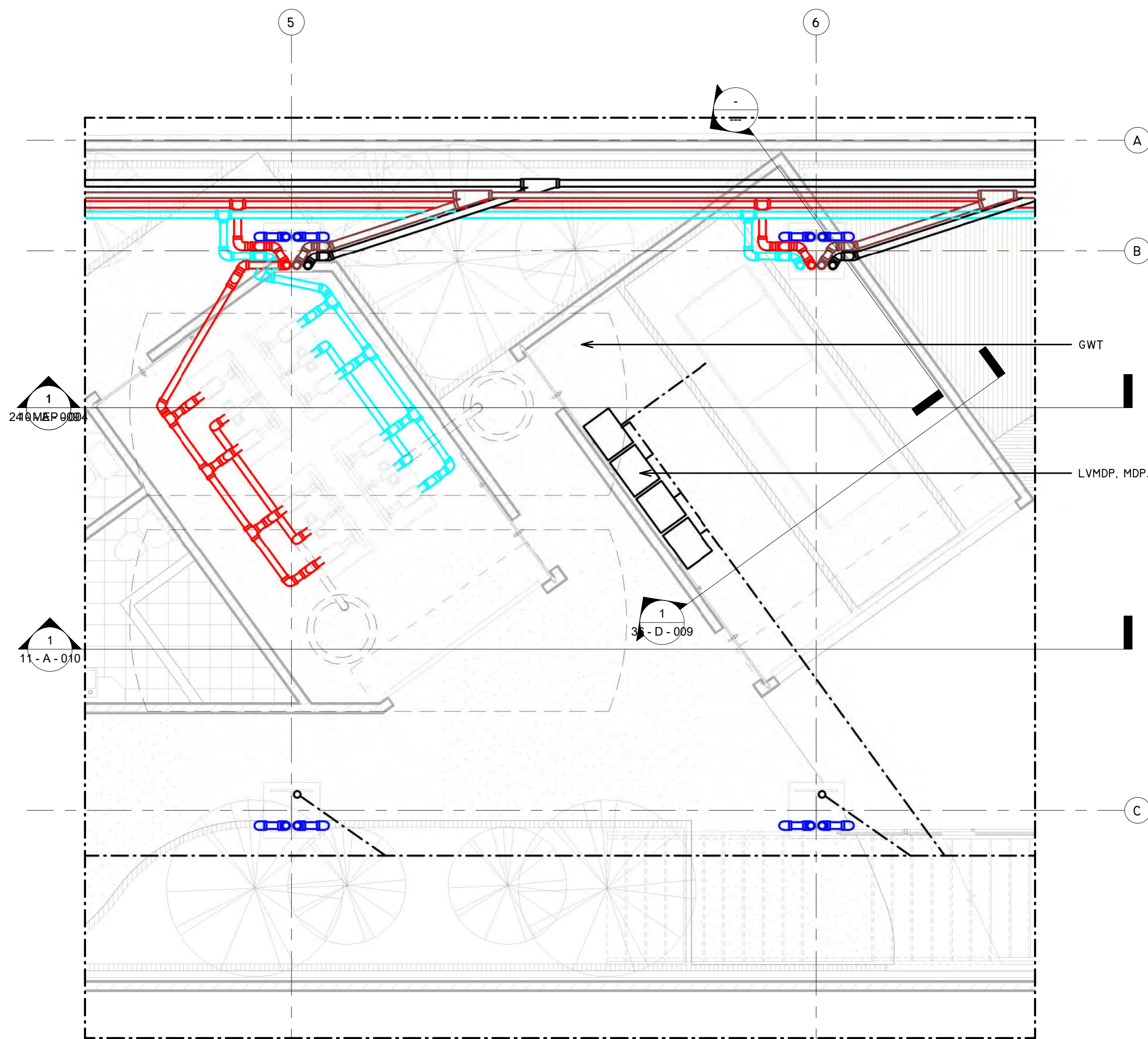
GROUND FLOOR - SKEMA SISTEM PENYEDIAAN AIR BERSIH - DETAIL DISTRIBUSI AIR, LIMBAH DAN ENERGI
