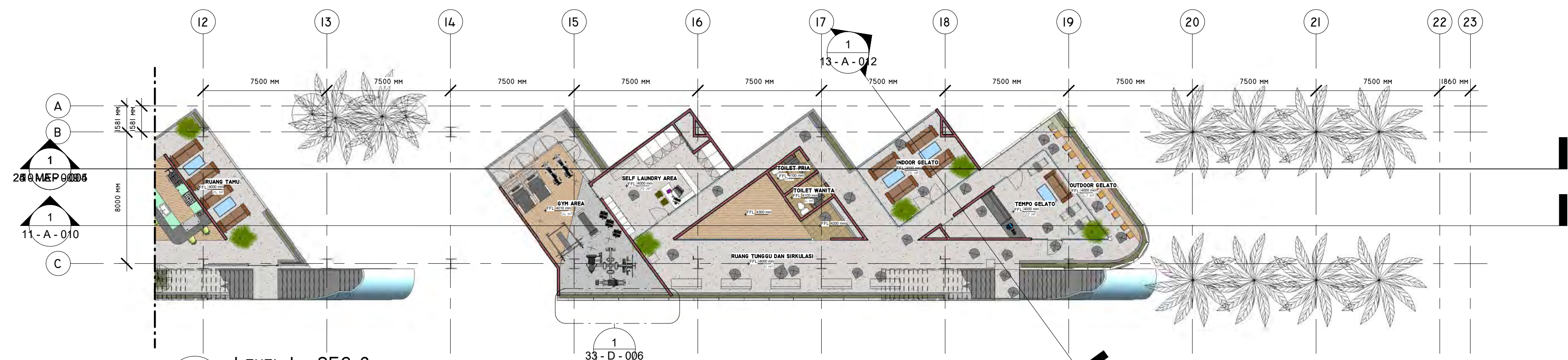
2 05 - A - 004 1 : 200 LEVEL I - SEC 2
