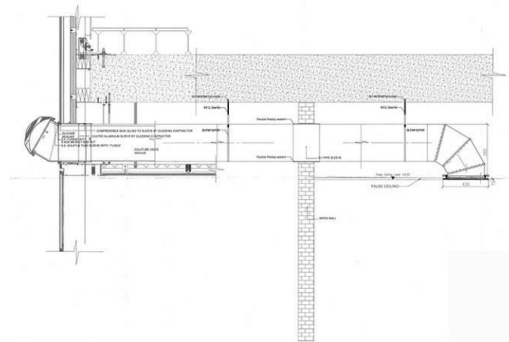
Gambar 2. 29 Light Pipe sebagai pendistribusi cahaya alami (Sumber: www.archsd.gov.hk )
