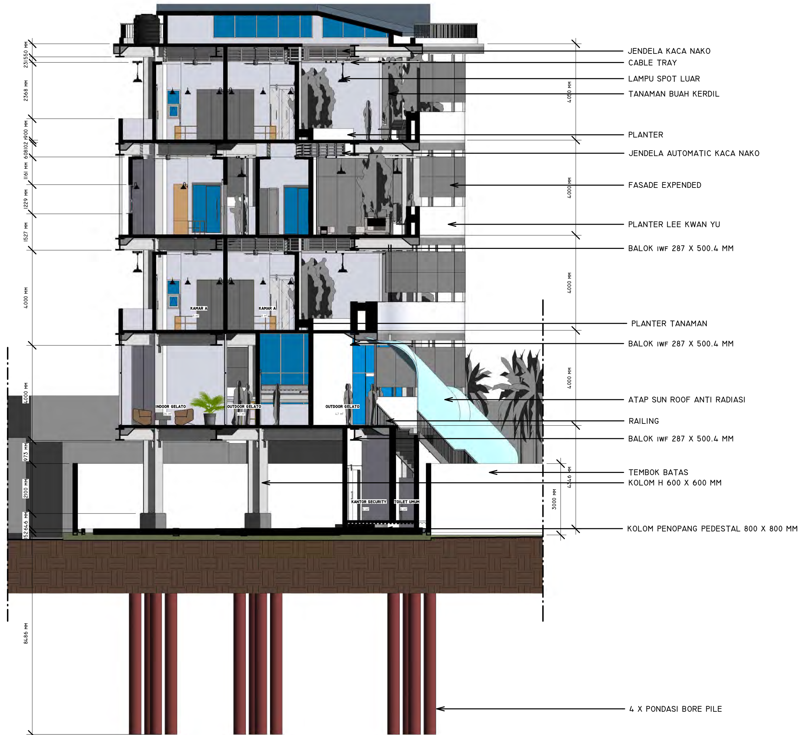
SECTION D-D 13 - A - 012 1 : 100
