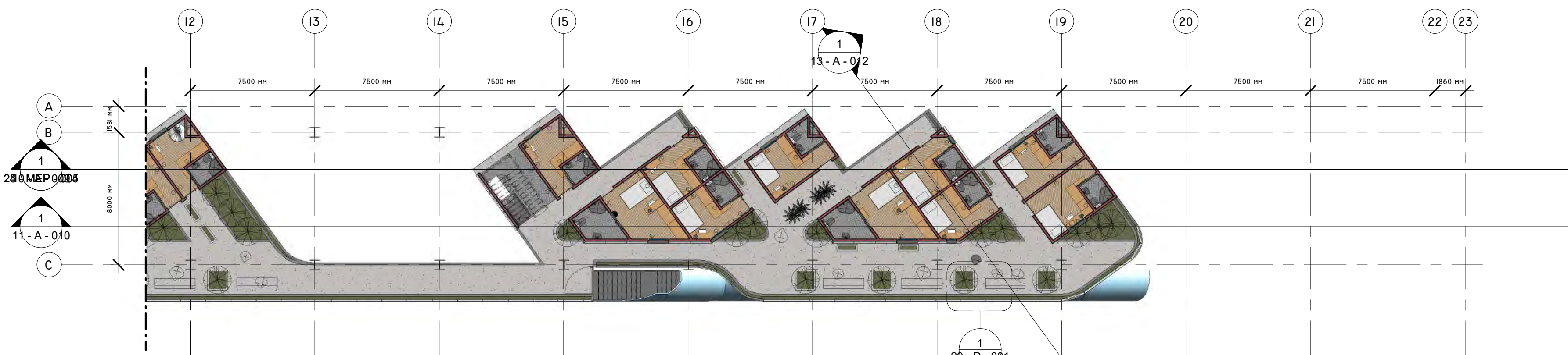
2 08 - A - 007 LEVEL 4 - SEC 2 1 : 200
