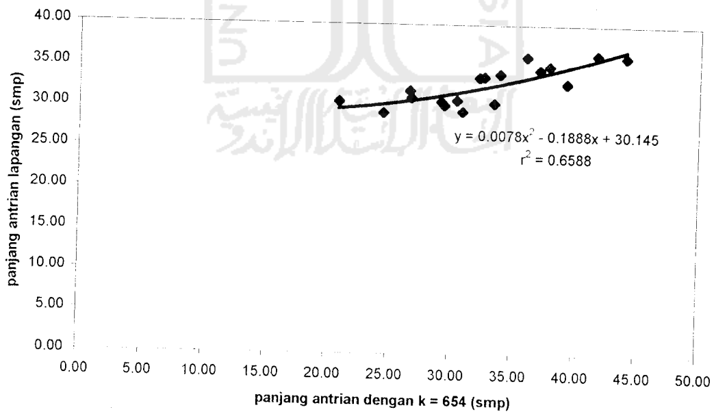
Gambar 5.8 Regresi polinomial panjang antrian lapangan dan k = 654
