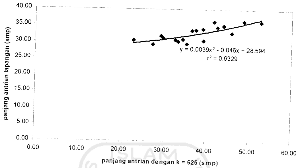
Gambar 5.7 Regresi polinomial panjang antrian lapangan dan k = 625
