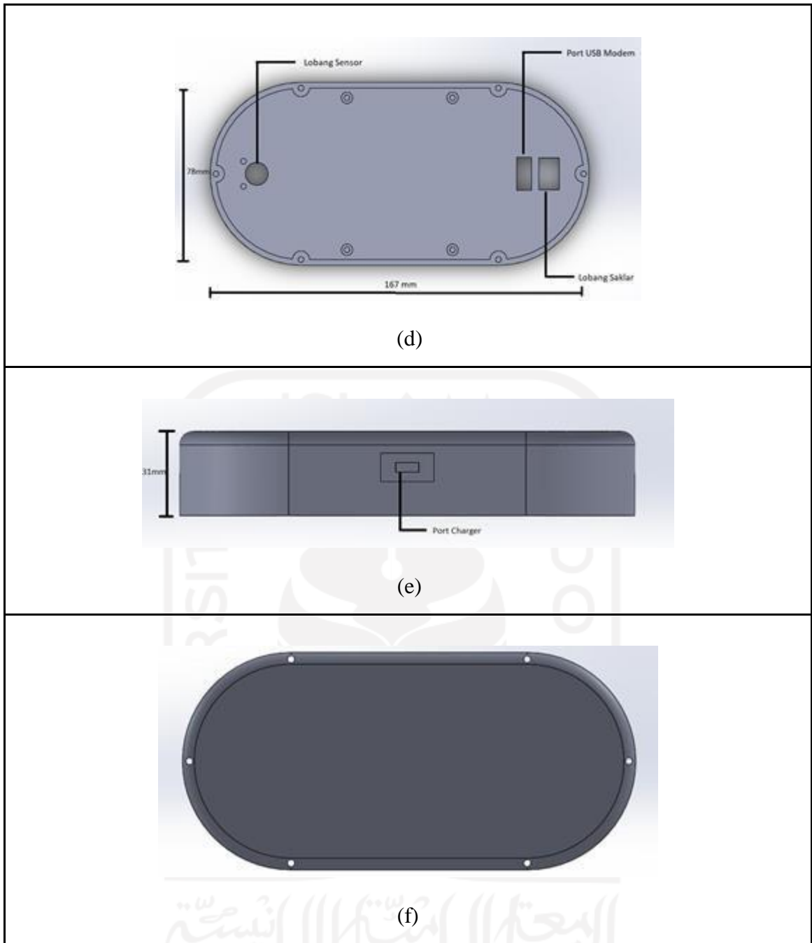
Gambar 4.1. Perbandingan bentuk case rancangan awal dan realisasi (a) desain lama tampak depan. (b) desain lama tampak belakang. (c) desain baru tampak atas. (d) desain baru tampak samping. (e) desain baru tampak dalam. (f) desain baru tampak dalam.
