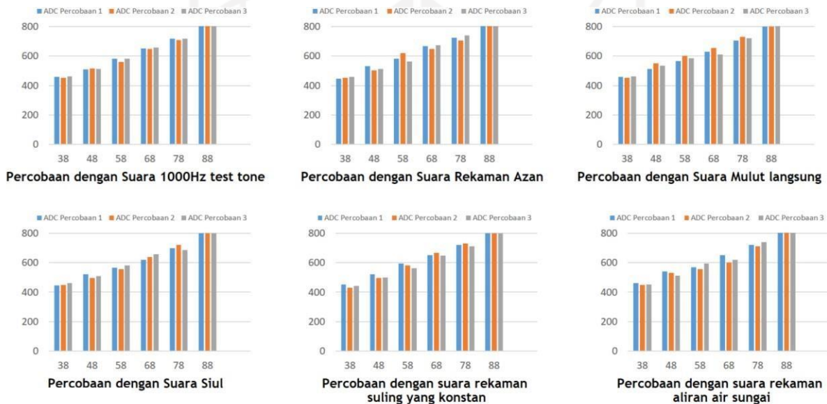
Gambar 5.1 Hasil perbandingan nilai ADC beberapa sampel suara
