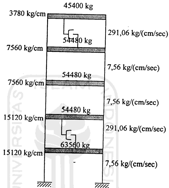
Gambar 4.15 Struktur dengan posisi MR dampers pada tingkat kedua dan kelima
