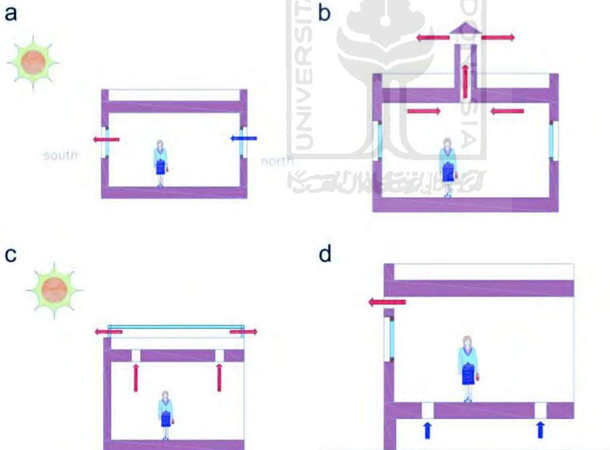
Gambar Alternatif Ventilasi Ruang Sumber : (Manzano-Agugliaro, Montoya, Sabio-Ortega, & García-Cruz, 2015)
