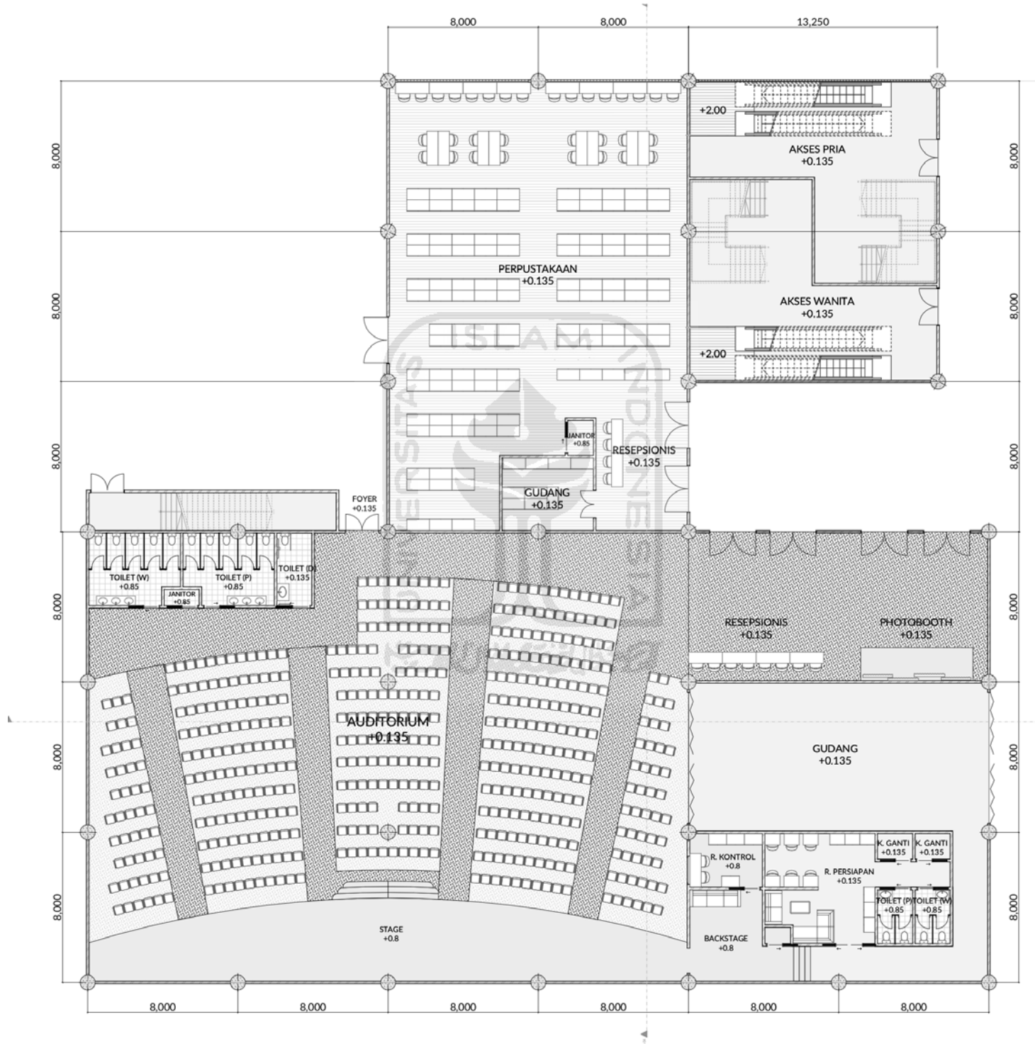
Gambar 74. Denah Lt. 1 alternatif desain 01 Sumber : Hernanta, 2020
