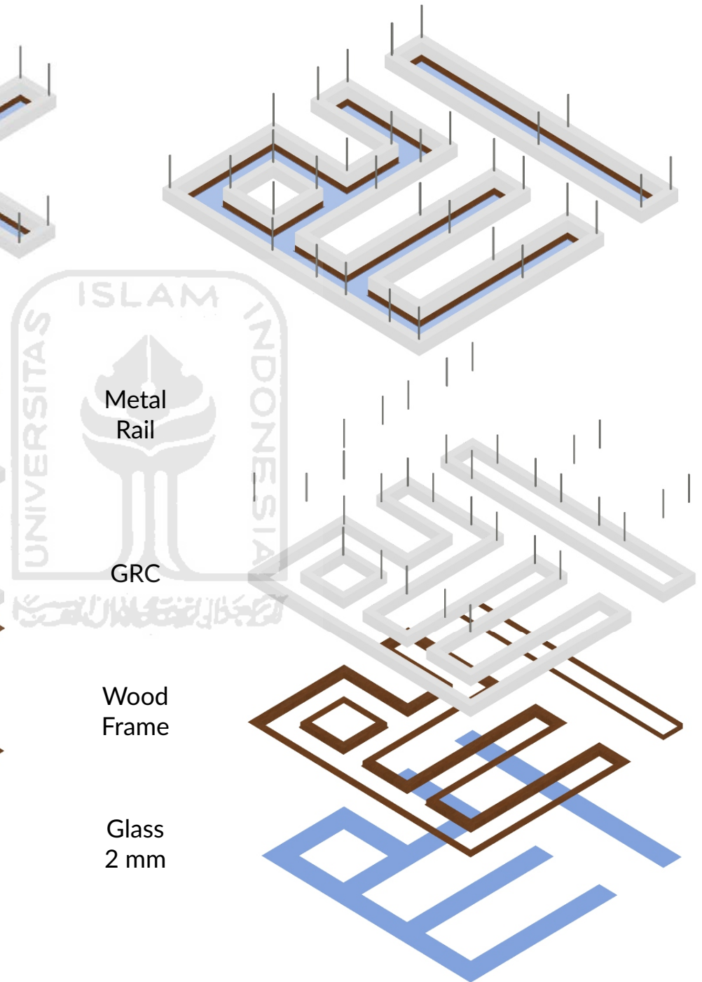
Gambar 134. (Kanan) Exploded fasad bangunan utama Sumber : Hernanta, 2020
