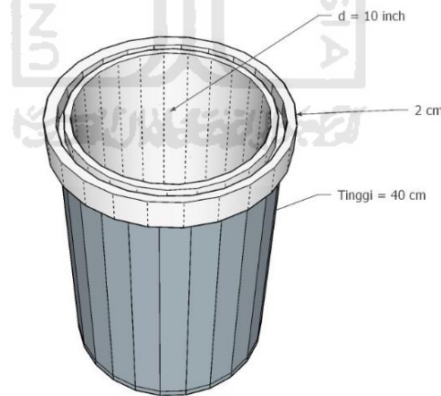
Gambar 2 Chamber tampak dalam
