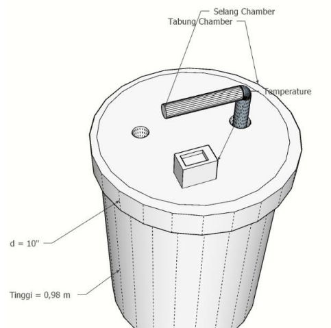
Gambar 3 Chamber Tampak Atas
