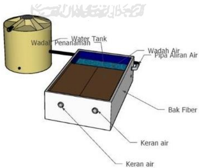
Gambar 8 Rangkaian Alat Penanaman Tampak Depan
