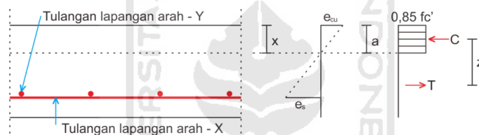
Gambar 3.4 Penulangan Pelat Daerah Lapangan
