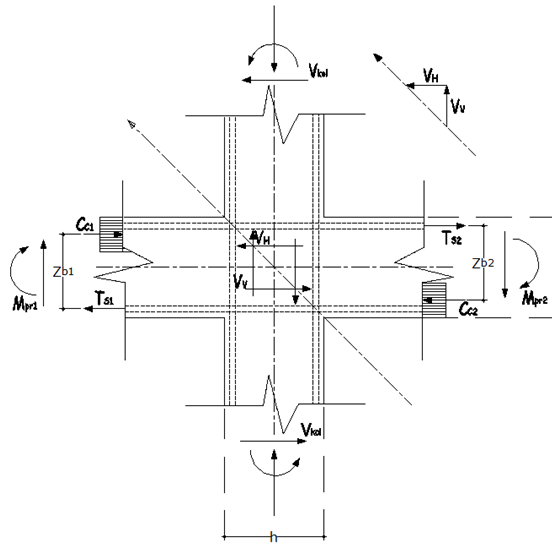
Gambar 3.8 Gaya-gaya pada Hubungan Balok Kolom
