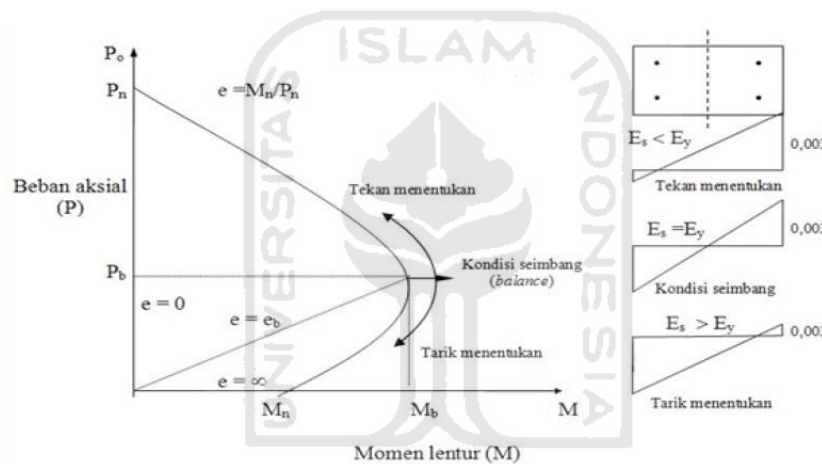
Gambar 3.7 Diagram Interaksi Kolom P dan M
