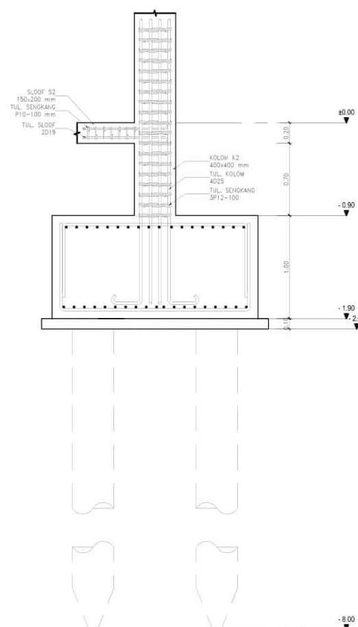
PONDASI P2 1:50
