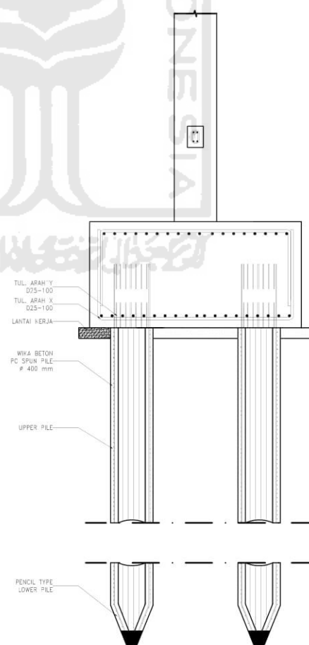
POTONGAN B-B PONDASI P2 1:50
