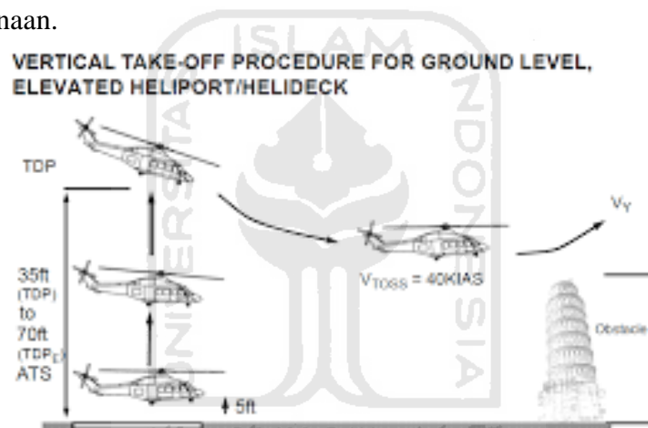
Gambar 5.22 Parameter Ketinggian Helikopter Lepas Landas
