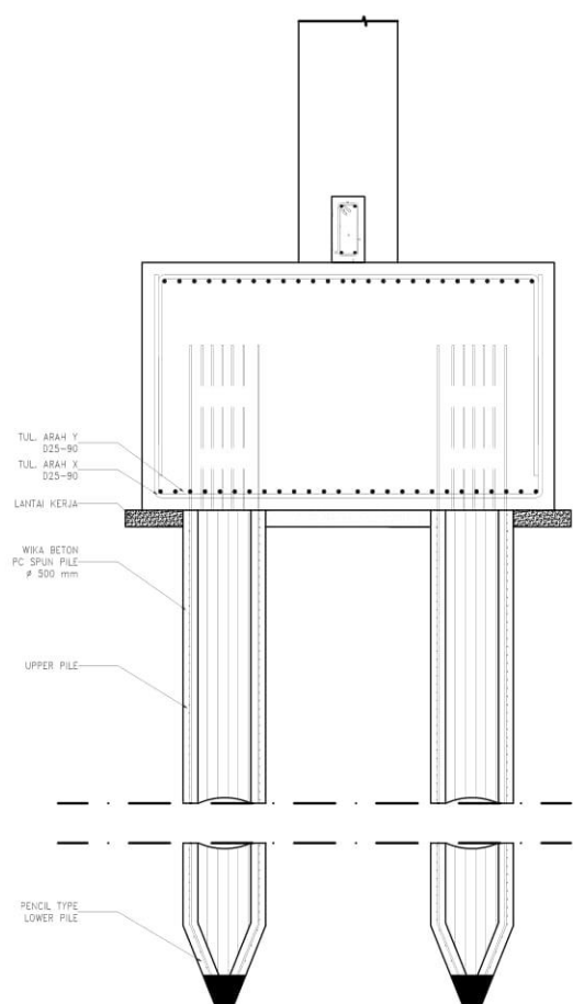
POTONGAN B-B PONDASI P1 1:50
