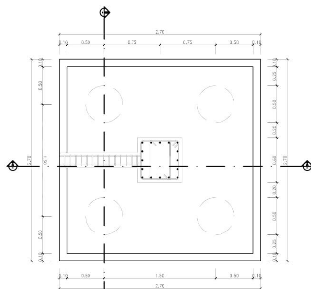
PONDASI P1 1:50
