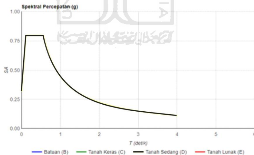
Gambar 3.2 Respon Spektrum pada Lokasi yang Ditinjau
