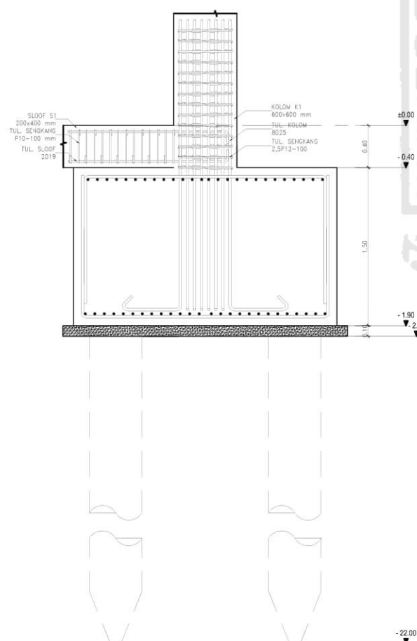
PONDASI P1 1:50
