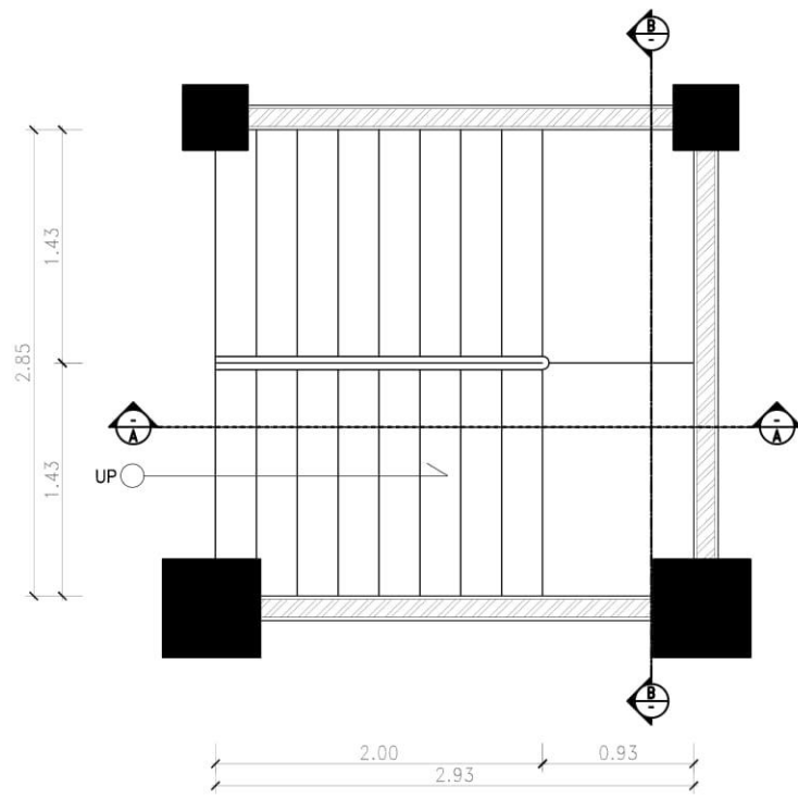
DENAH TANGGA LANTAI 2-3 1:50
