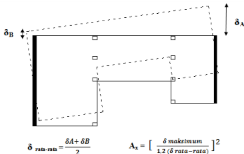
Gambar 5.3 Ketidakberaturan Torsional 1a dan 1b
