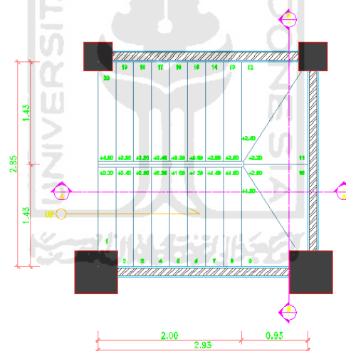
Gambar 5.13 Denah Tangga Lantai 1
