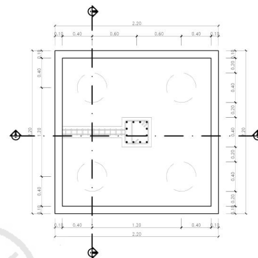
PONDASI P2 1:50
