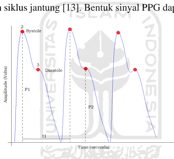
Gambar 2.2 Sinyal PPG Sistol dan Diastol [14].
