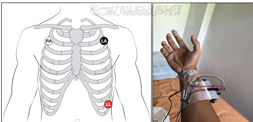
Gambar 3.4 Peletakan EKG pada Dada (Kiri) [20], PPG pada Ujung Jari Telunjuk Kanan dan Pergelangan Tangan Kanan (Kanan)
