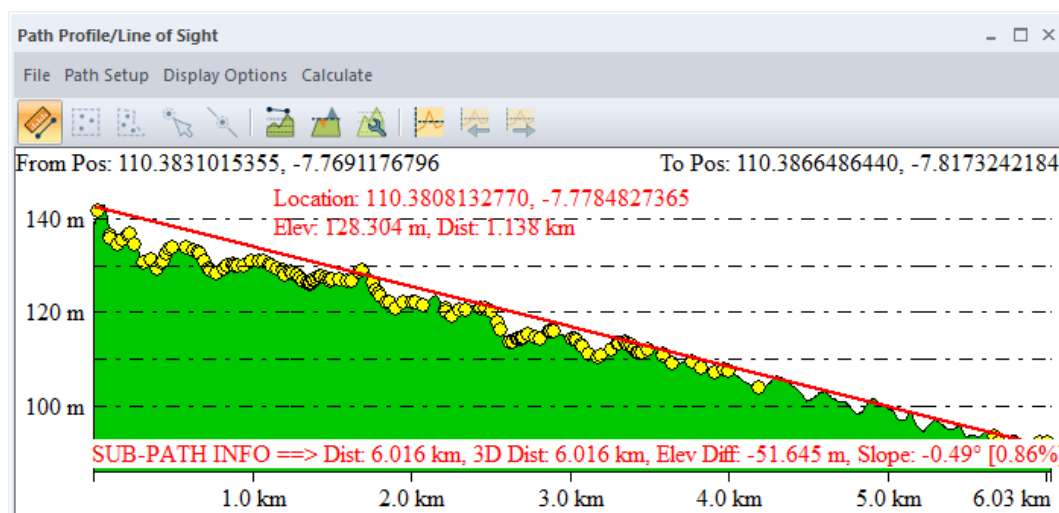
Gambar 5.14 Beda elevasi dan panjang Kali Belik Melalui Aplikasi Global Mapper
