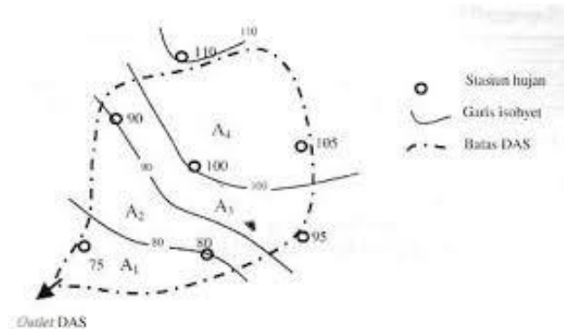
Gambar 3.7 Metode isohyet
