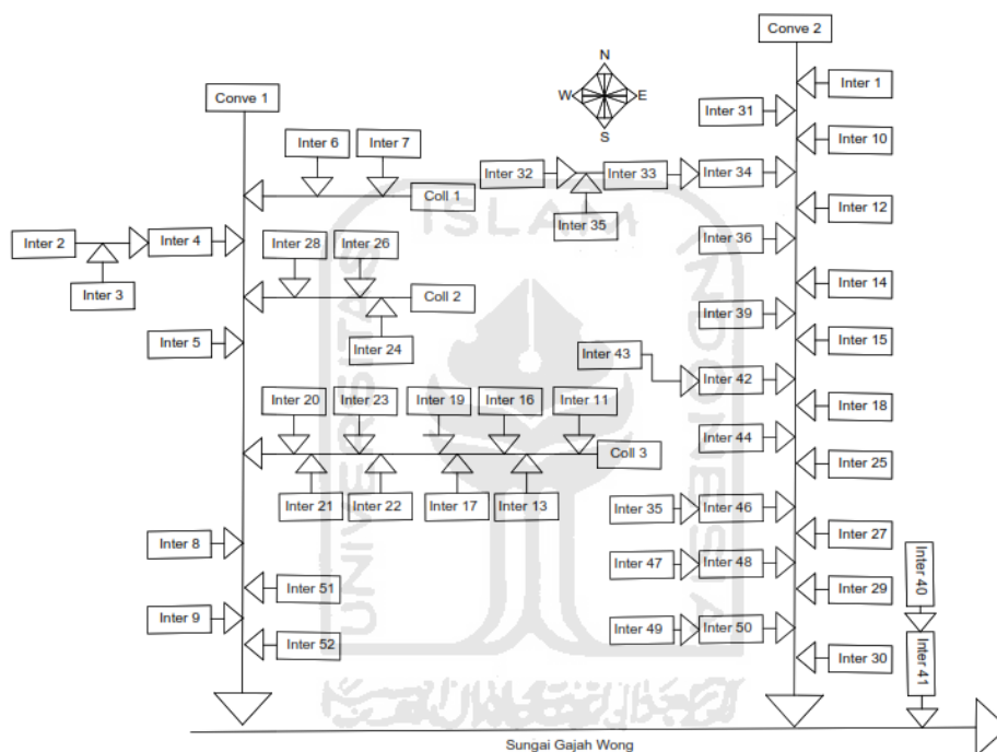
Gambar 5.2 Skema dan Arah Aliran Saluran Drainase
