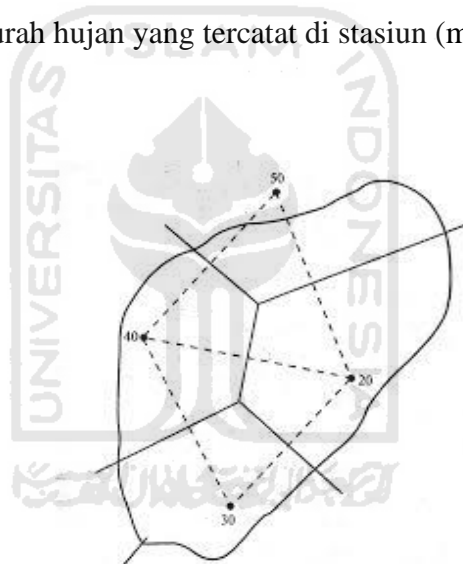
Gambar 3.6 Metode Poligon Thiessen
