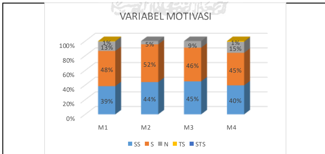
Gambar 4. 10 Persentase Persebaran penilaian parameter Motivasi
