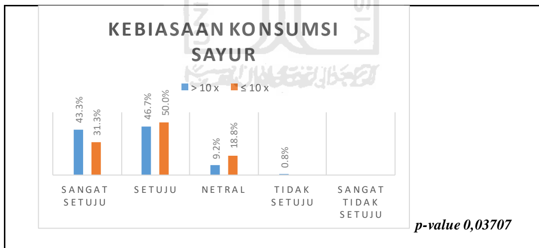
Gambar 4. 14 Hubungan Antara Indikator M1 (kebiasan konsumsi sayur) terhadap Intensitas Pembelian
