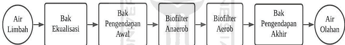
Gambar 13. Tahapan Pengolahan Air Limbah Proses Kombinasi Biofilter Anaerob-Aerob
