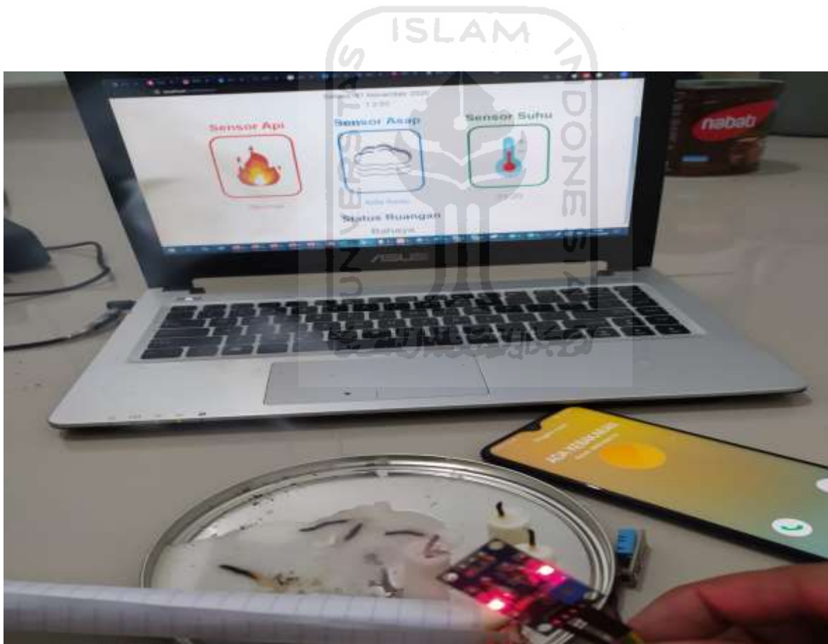
Gambar 4.13 Pengujian sensor asap
