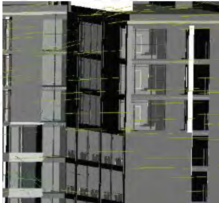
Gambar 4.7 Simulasi Angin pada Koridor Apartemen Timur ke Barat
