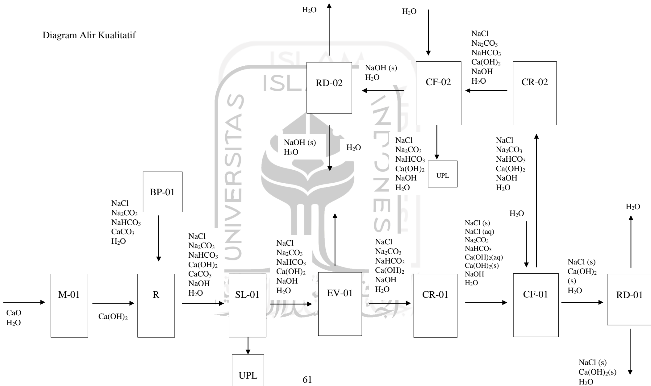
Gambar 4. 3 Diagram Alir Kualitatif
